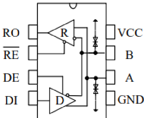
图 1 ES3485EEUA 引脚分布图
