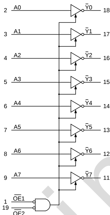
图 1 逻辑符号
