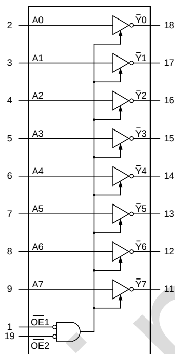
图 3 功能框图
