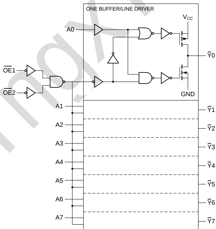
图 4 逻辑框图
