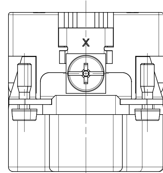
C146 M Rahmen mit 3 Steckplätzen frame with 3 slots
