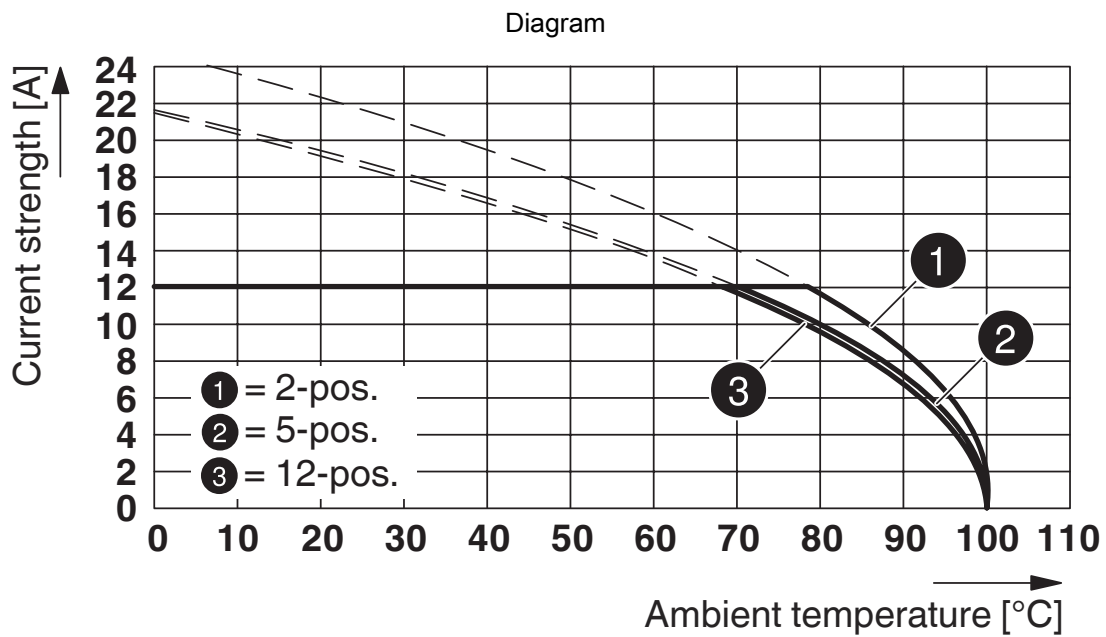
Type: GIC 2,5/...-ST-7,62 with GICV 2,5/...-G-7,62
