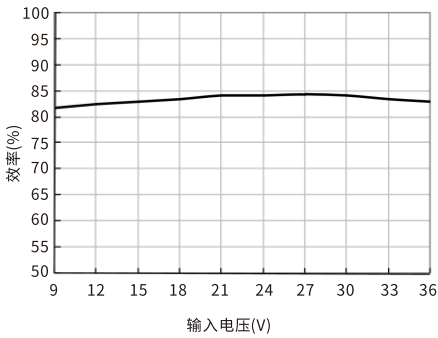
效率Vs输入电压(满载) URB2405YMD-10WR3
