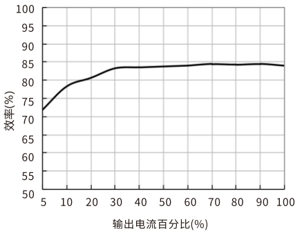
效率Vs输出负载(Vin=24V) URB2405YMD-10WR3
