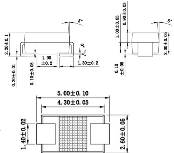
SMA(DO-214CA)
