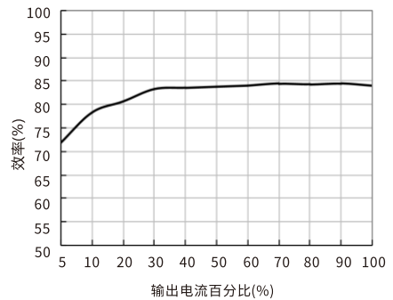
效率Vs输出负载(Vin=24V) URB2405YMD-15WR3
