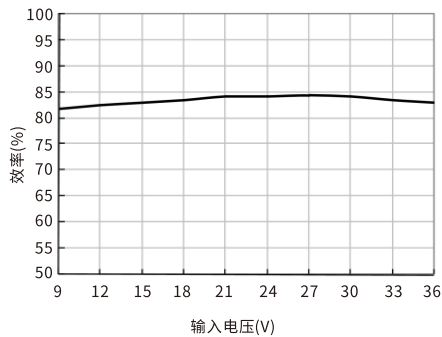
效率Vs输入电压(满载) URB2405YMD-15WR3
