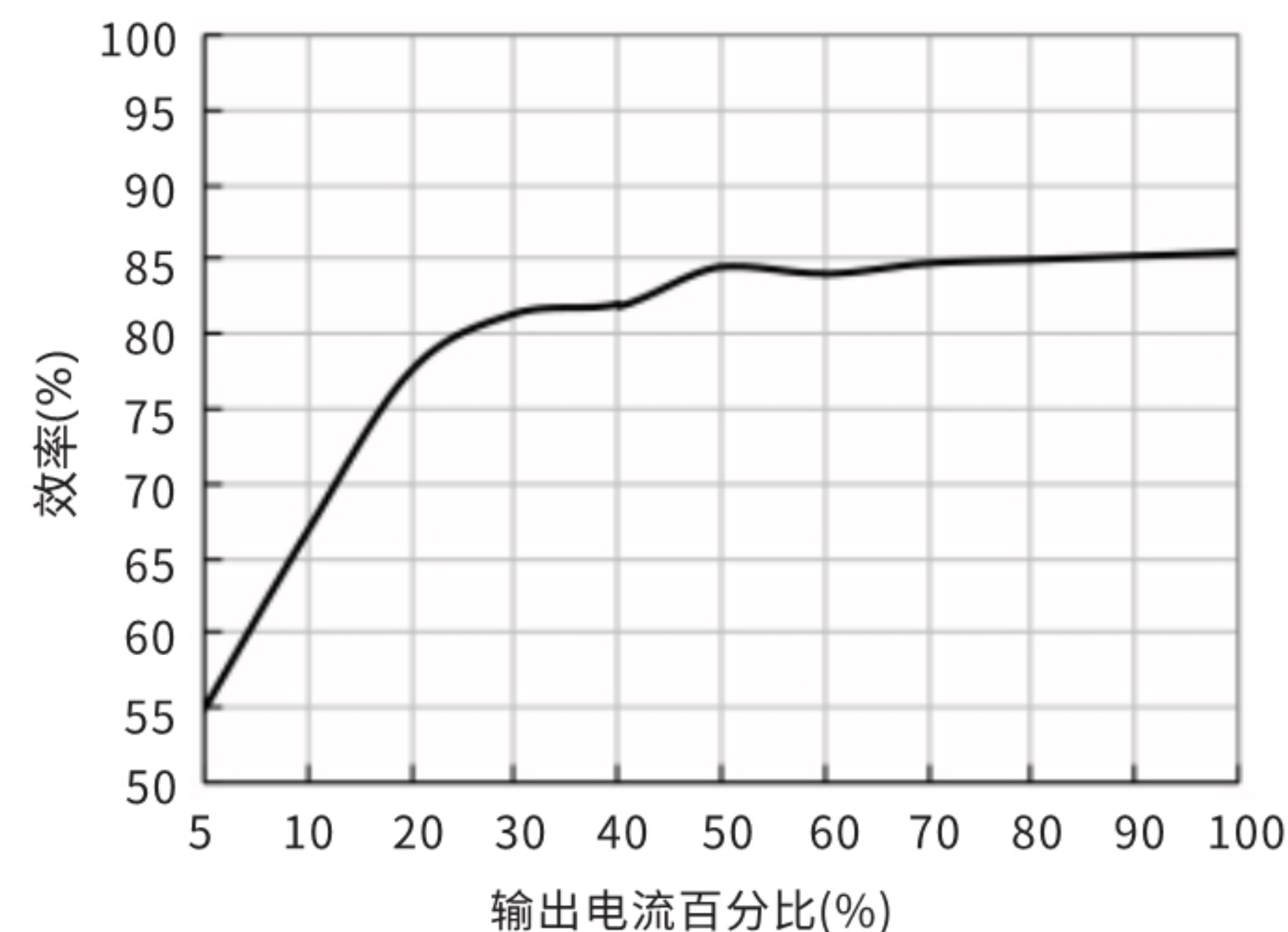
效率Vs输出负载(Vin=48V) URA4815YMD-6WR3
