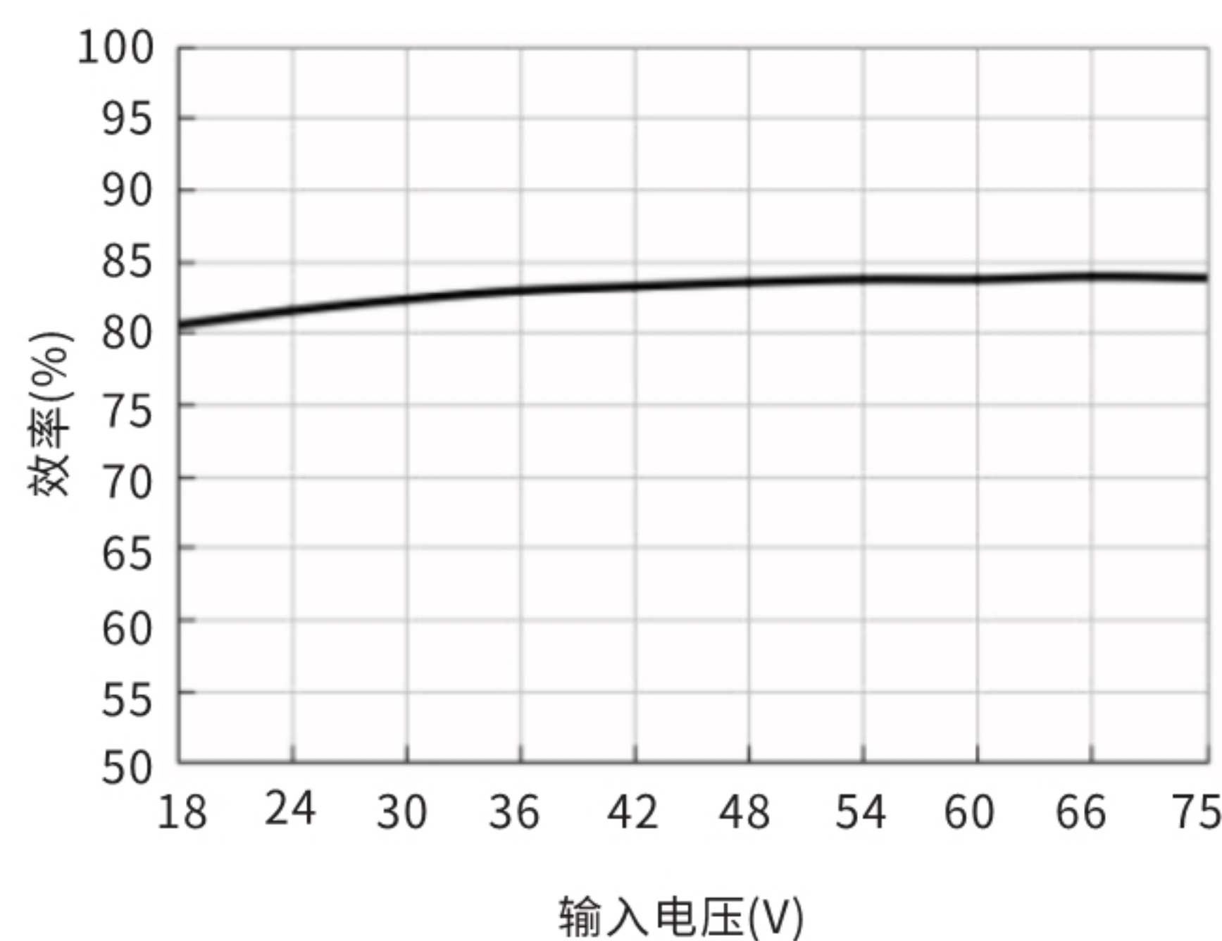
效率Vs输入电压(满载) URA4815YMD-6WR3
