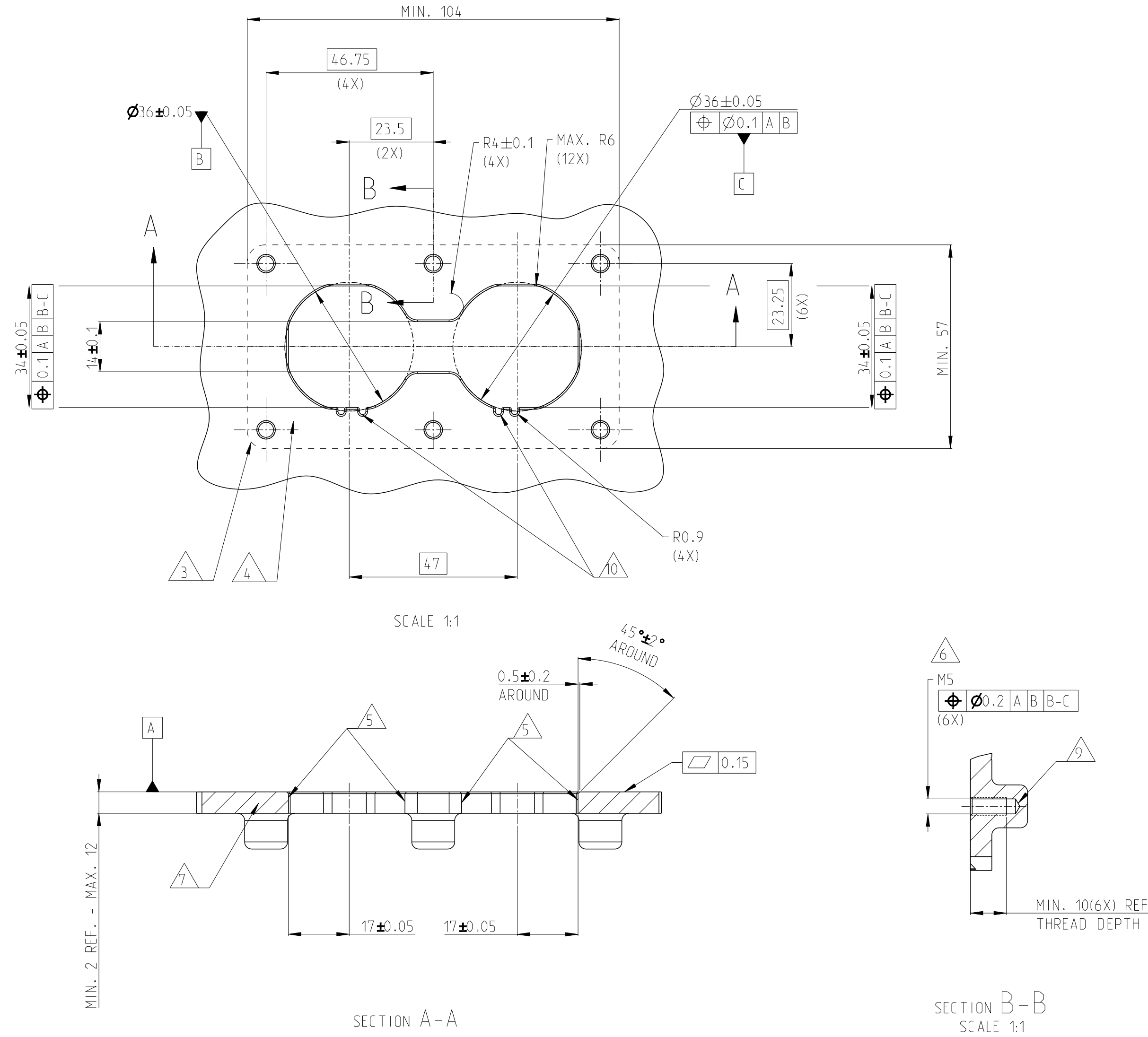
SECTION A-A
