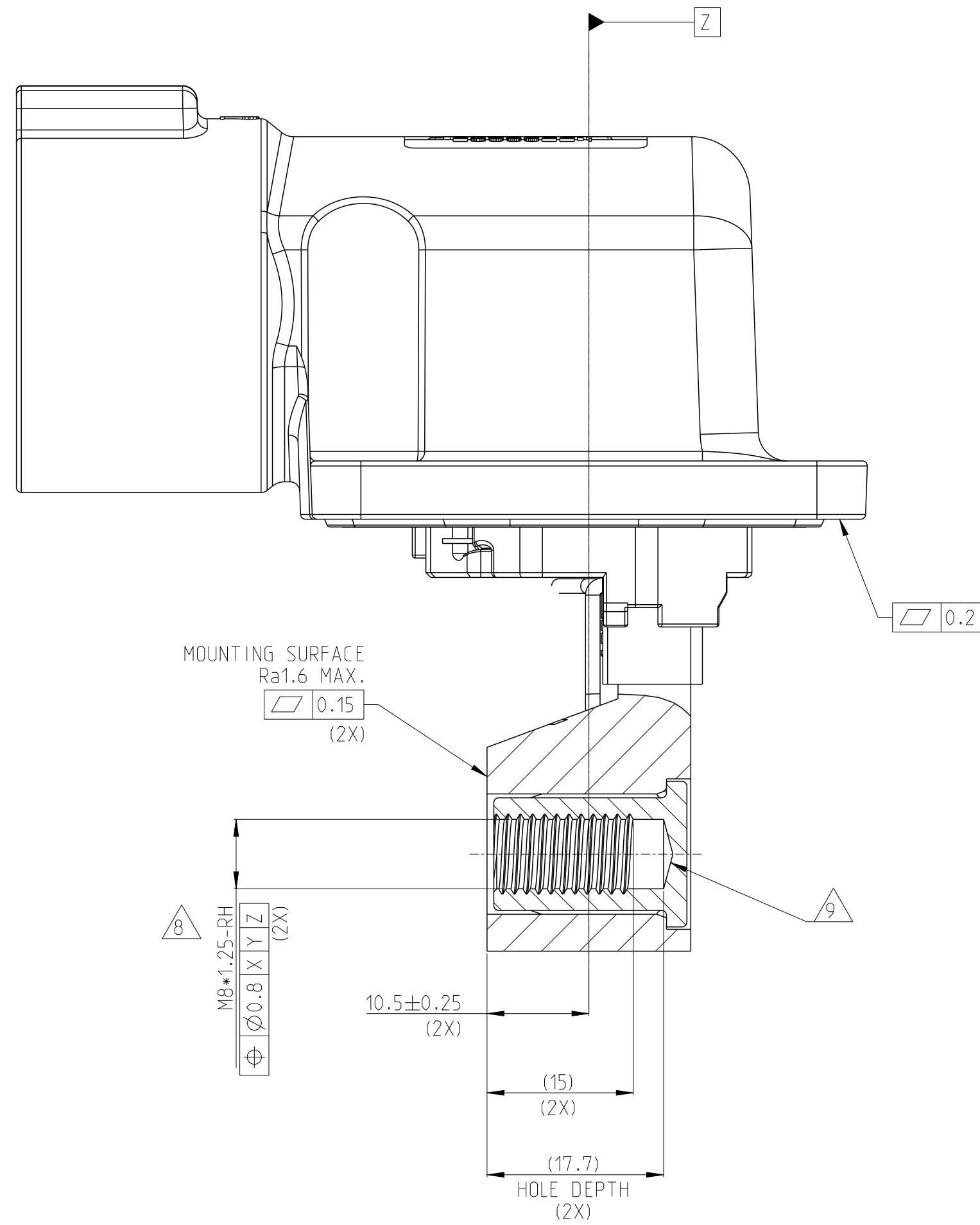
SECTION A-A
