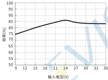
效率Vs输入电压(满载) URA2424S-6WR3
