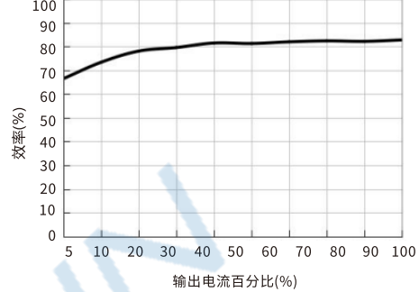
效率Vs输出负载(Vin=24V) URA2424S-6WR3
