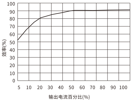
效率Vs输出负载(Vin=24V) URB2405YMD-20WR3
