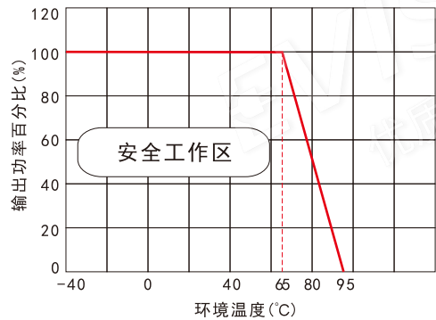
标称电压输入, 3.3V、5V输出 温度降额曲线图
