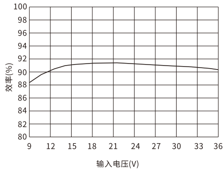
效率Vs输入电压(满载) URB2405YMD-20WR3
