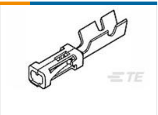
TE Part #2-87195-0 MOD IV RECP PLTD 30 DPLX
