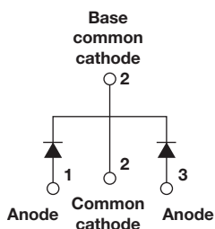
D 2 PAK (TO-263AB)
