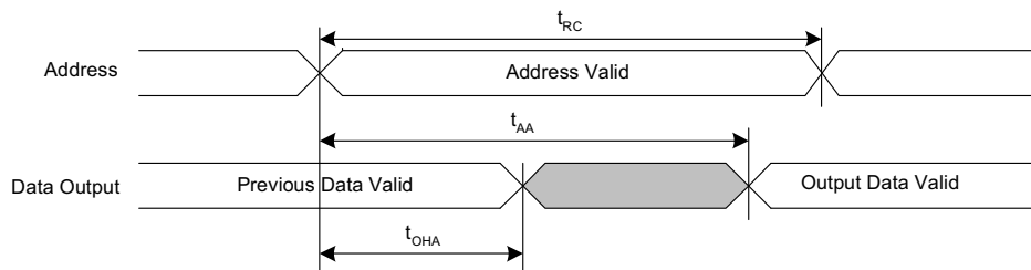
図 11. SRAM 読み出しサイクル 1: アドレス制御 [34、35、36]
