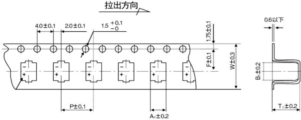
Fig.1 (Ø4 ~ Ø10)
