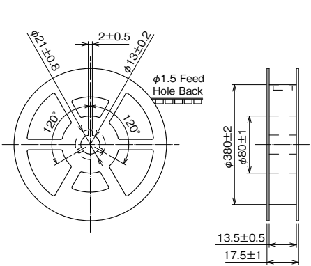
Reel Dimensions
