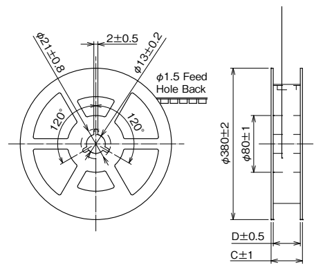
Reel Dimensions
