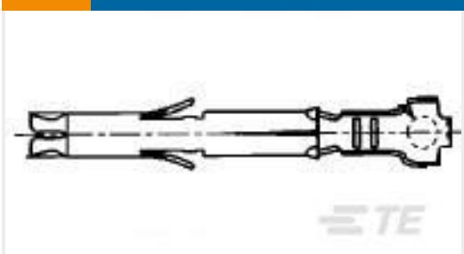
TE Part #170365-3 MINI UNIVERSAL M-N-L SOCKET LP
