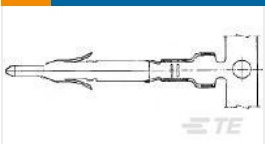
TE Part #170363-3 MINI UNIVERSAL M-N-L PIN LP
