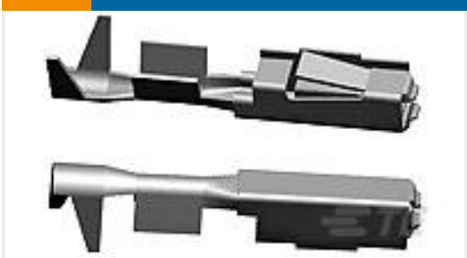
TE Part #5-968221-6 MOS0,63 Ag rec CB unseal. 0,5-0,75
