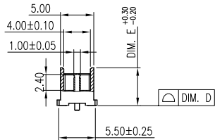
A-A SECTION
