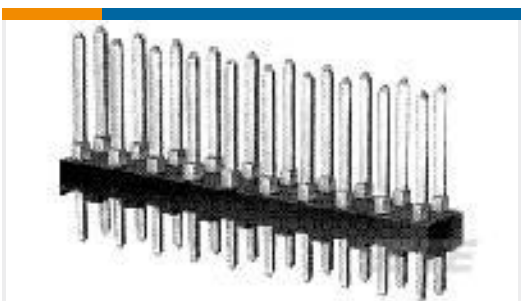
TE Part #1-87227-0 20 MODII HDR DRST UNSHRD .100
