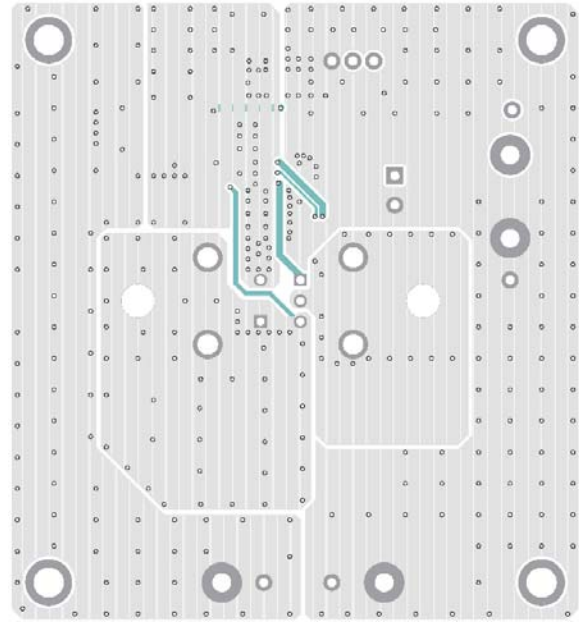
Figure 4—Bottom Layer
