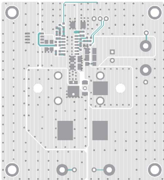
Figure 3—Top Layer
