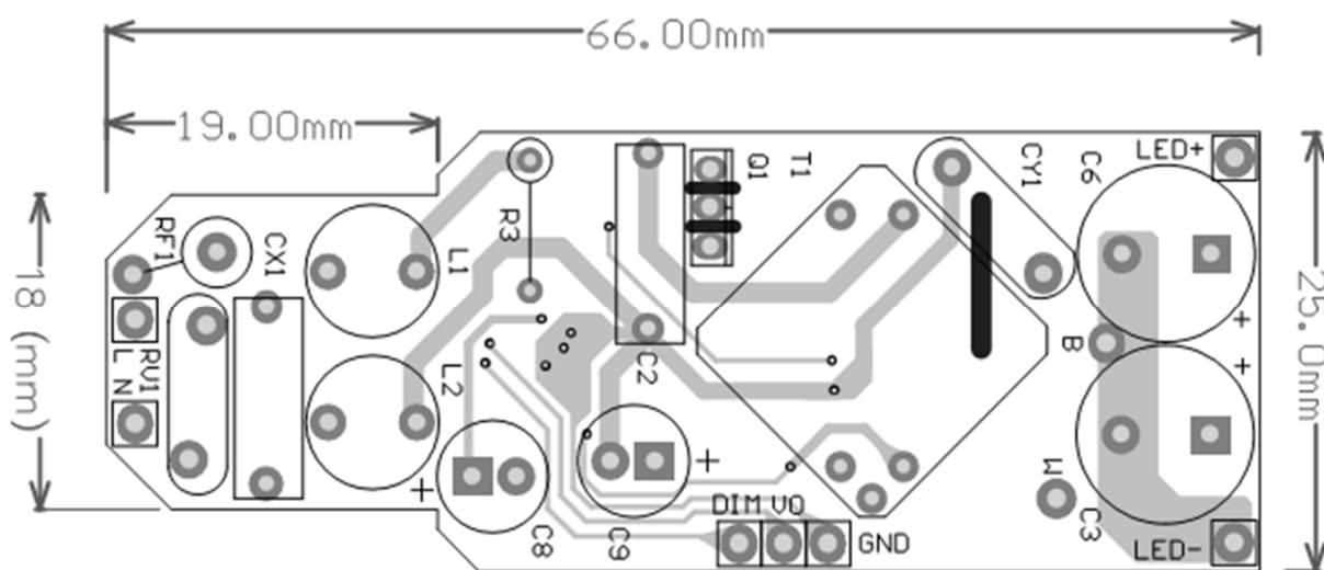
Bottom layer
