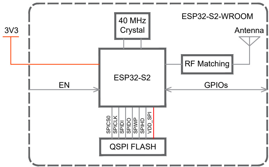
图 1: ESP32-S2-WROOM 功能框图
