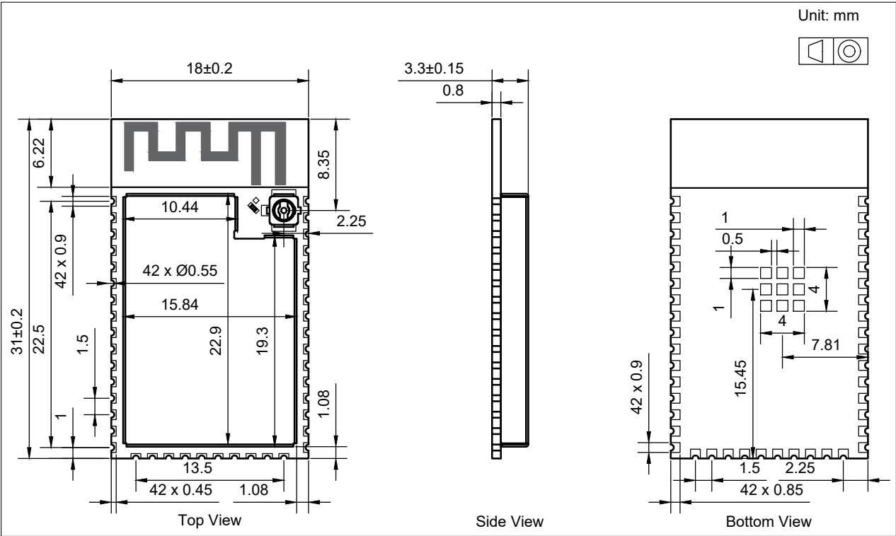
图 9: ESP32-S2-WROOM-I 模组尺寸
