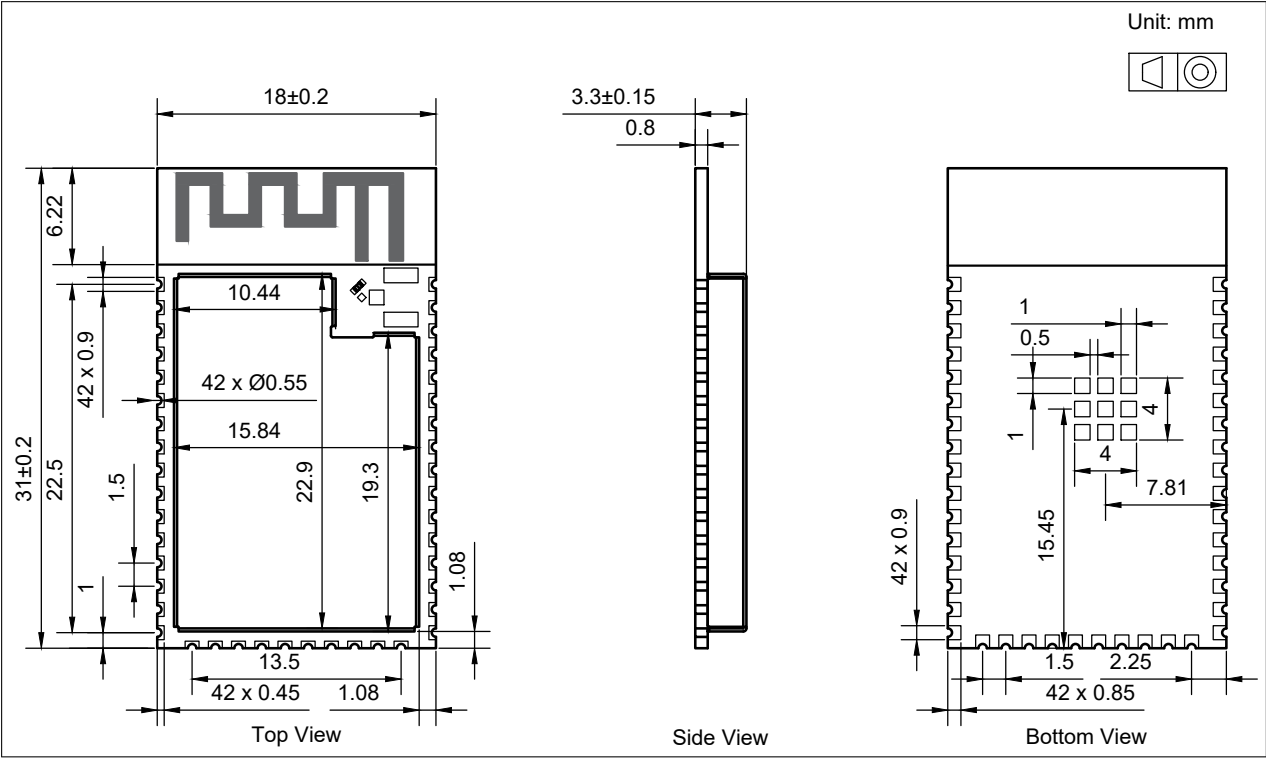
图 8: ESP32-S2-WROOM 模组尺寸
