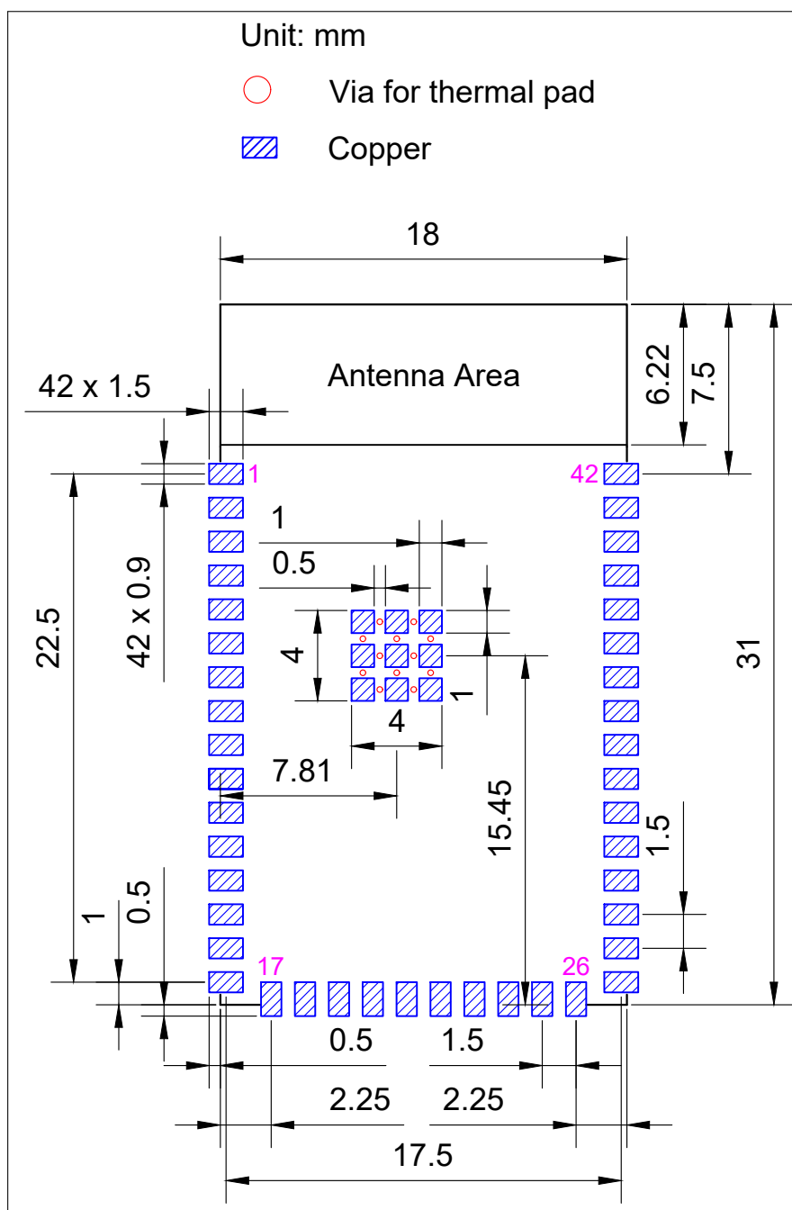
图 10: 推荐 PCB 封装图
