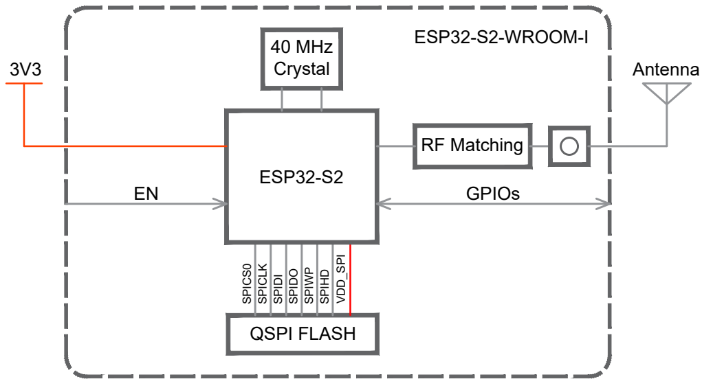
图 2: ESP32-S2-WROOM-I 功能框图
