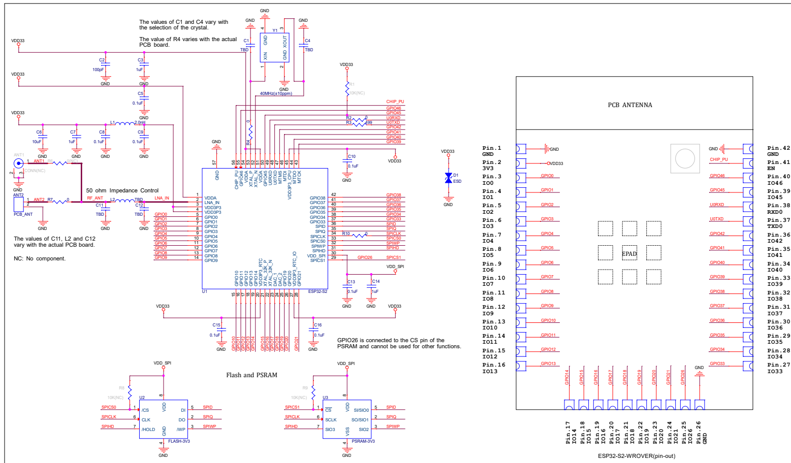
图 5: ESP32-S2-WROVER 原理图
