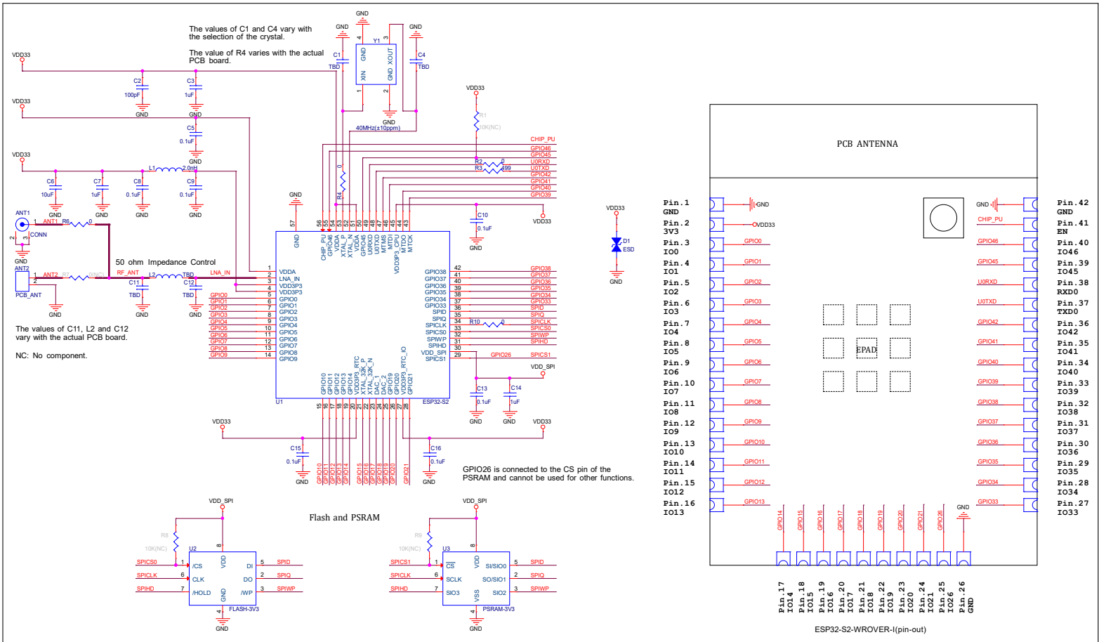
图 6: ESP32-S2-WROVER-I 原理图
