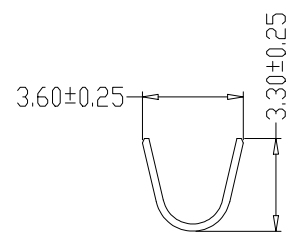
SBC-A-A
