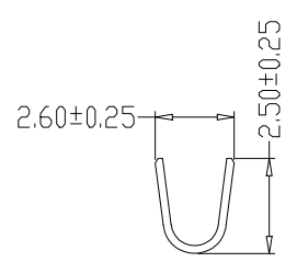
SBC-B-B
