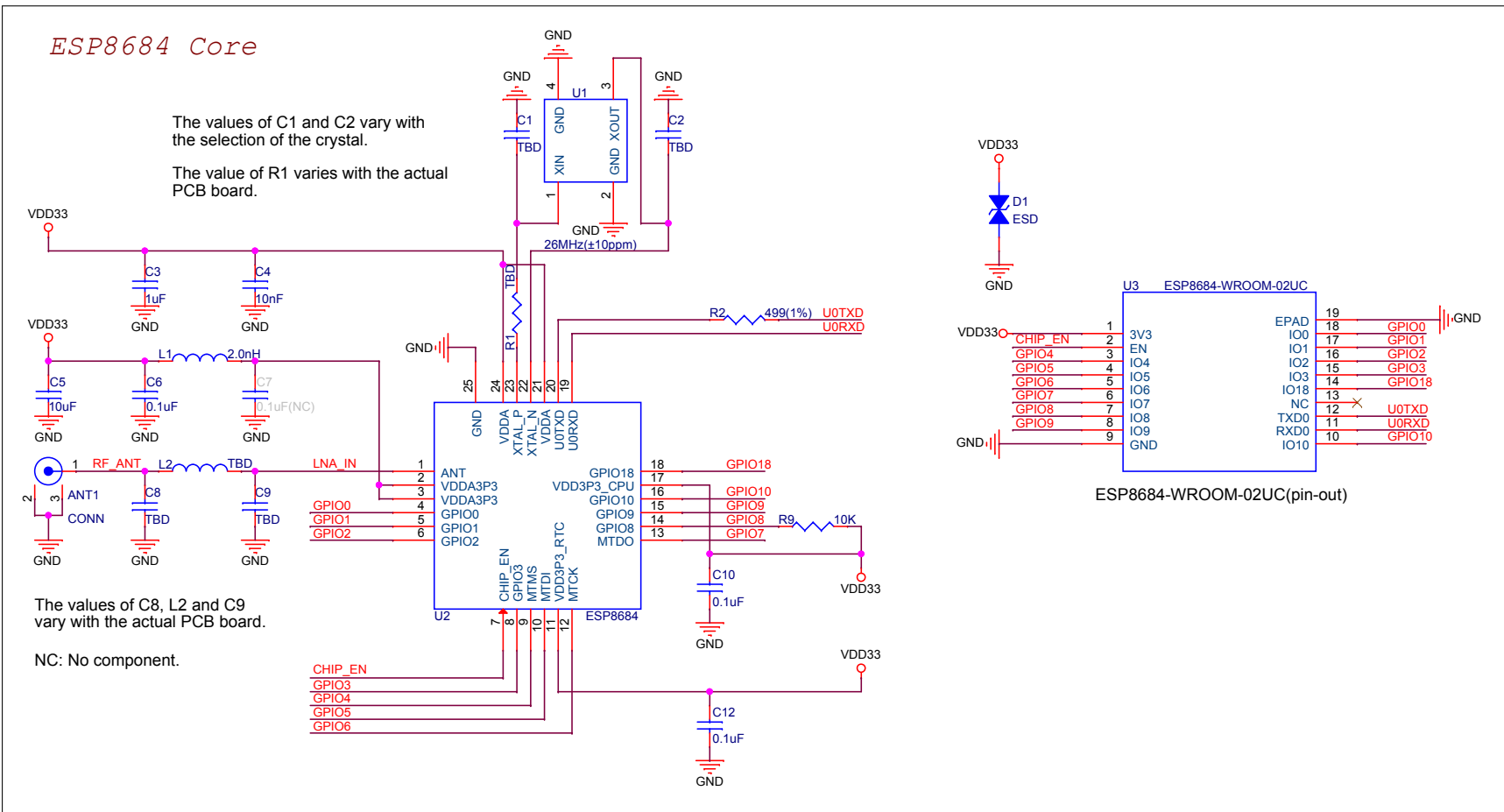
图 6: ESP8684-WROOM-02UC 原理图
