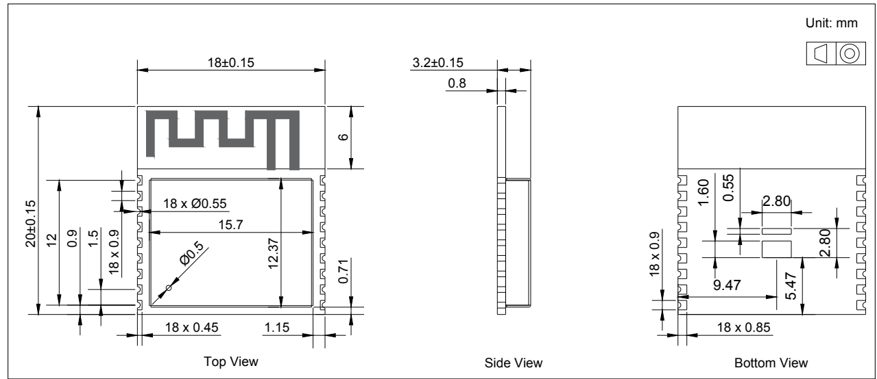
图 8: ESP8684-WROOM-02C 尺寸
