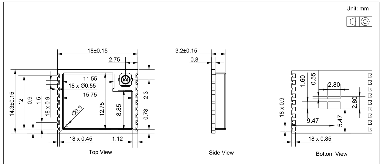
图 9: ESP8684-WROOM-02UC 尺寸
