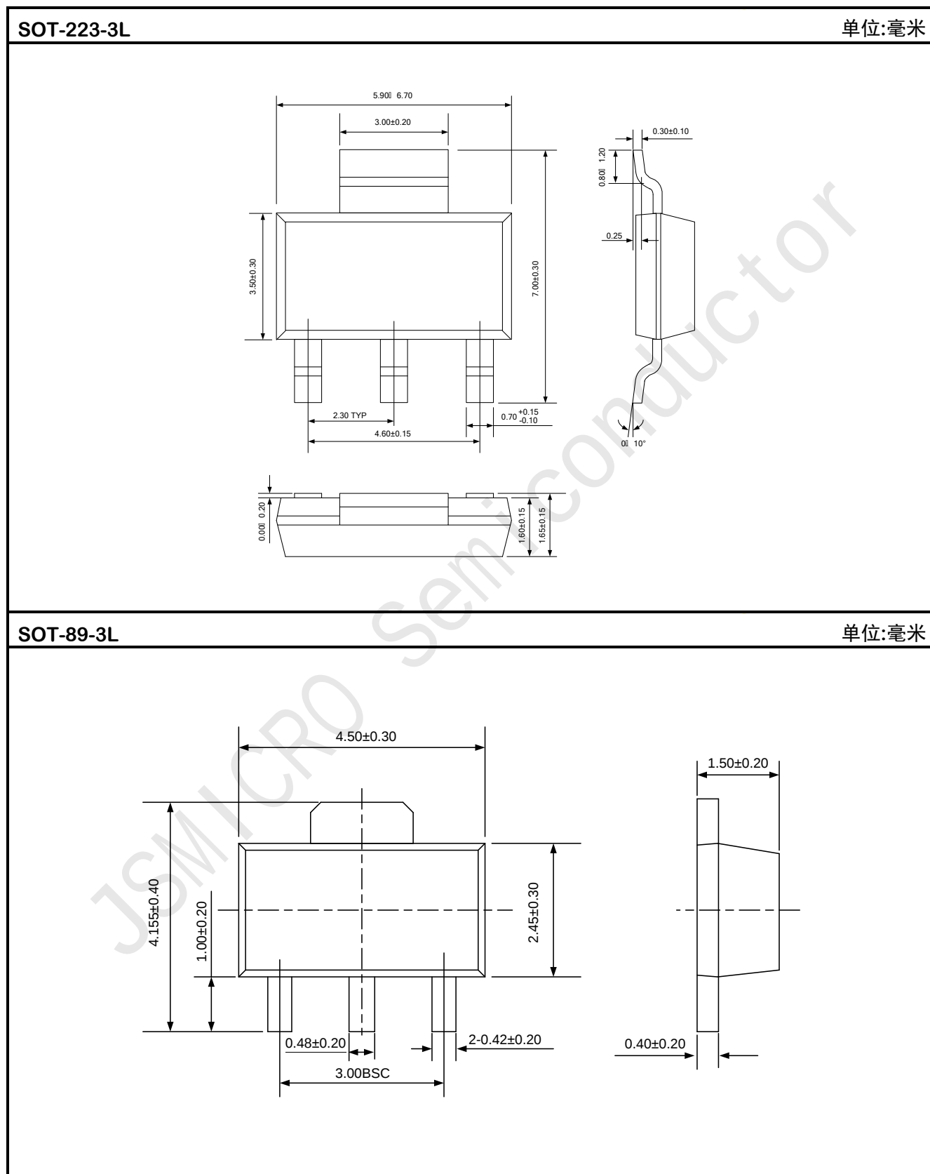
封装外形图
