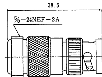
SJ-BNC(40)
