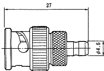
BNC-MSSJ(40)
