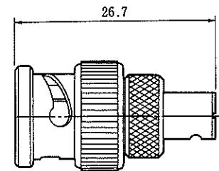
BNC-MSSP(40)
