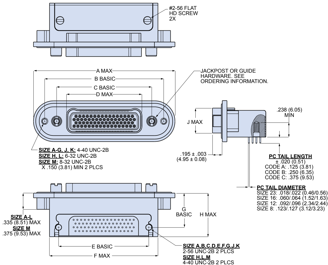
791-011P Dimensions
