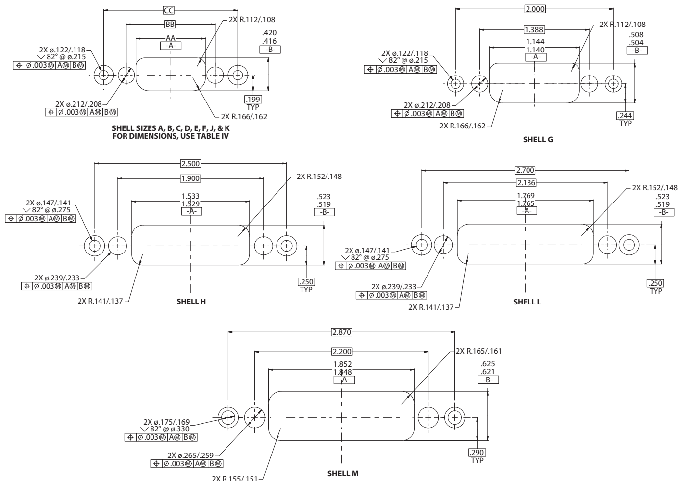
791-070 Dimensions
