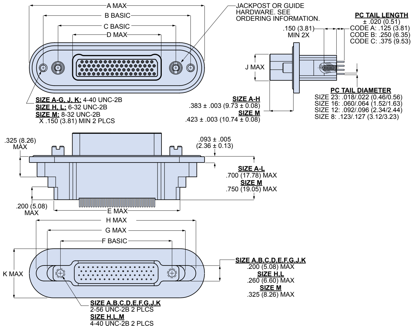
791-033S Dimensions
