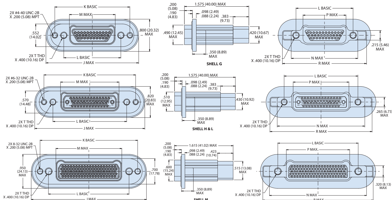
791-070 Dimensions
