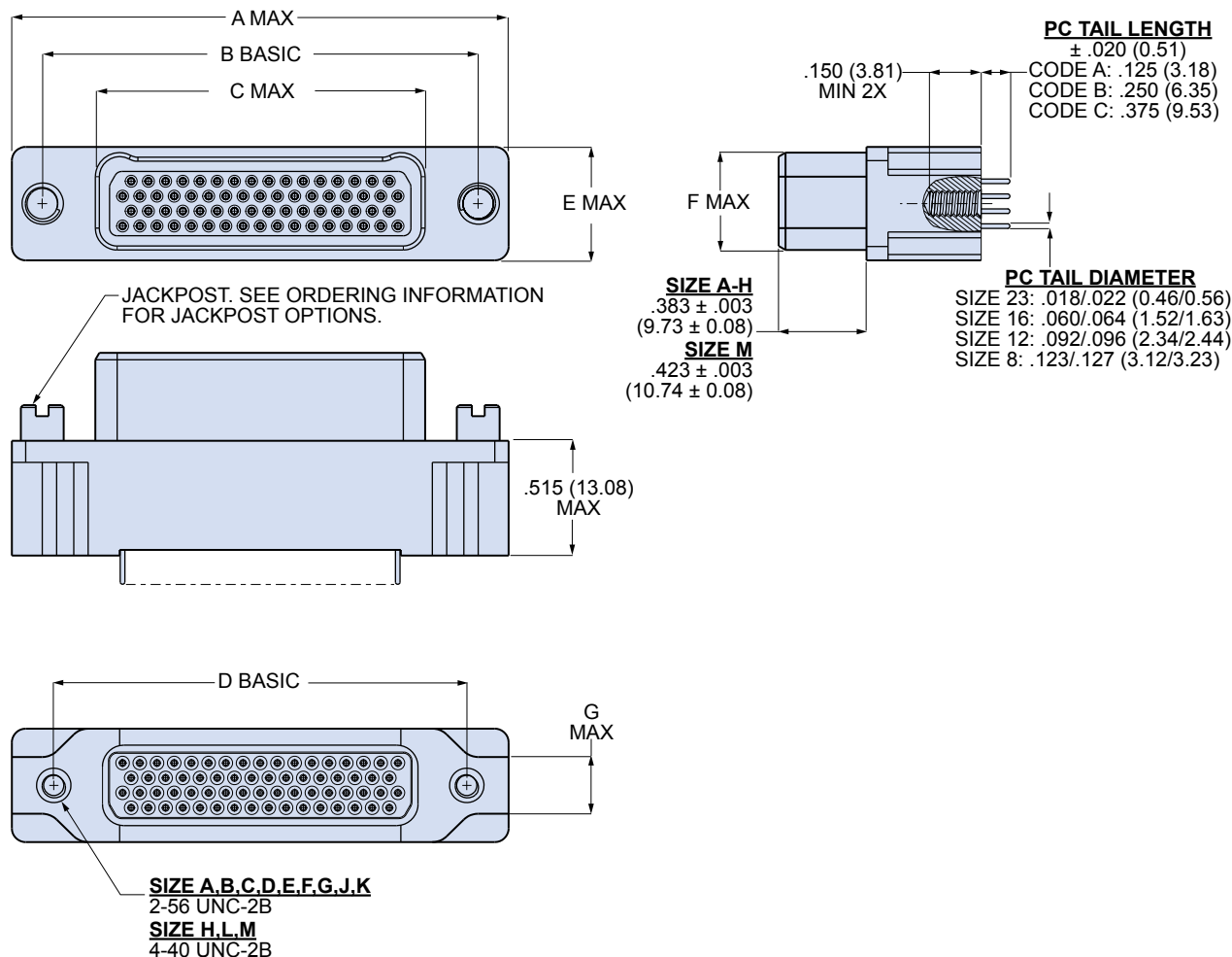
791-014S Dimensions
