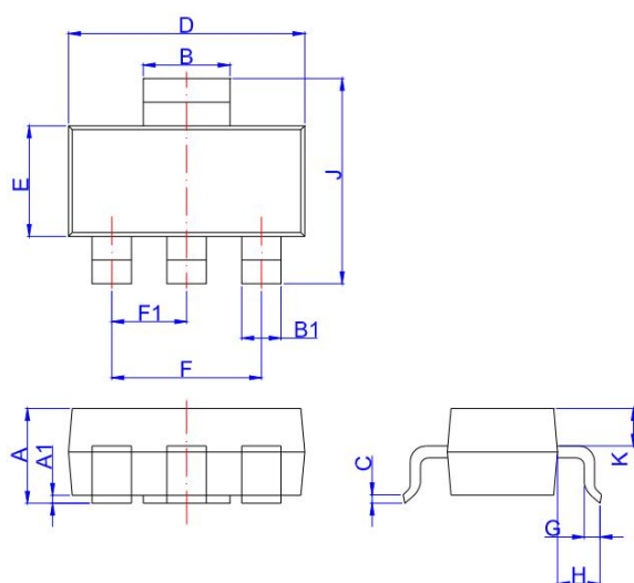
SOT-223-3L
