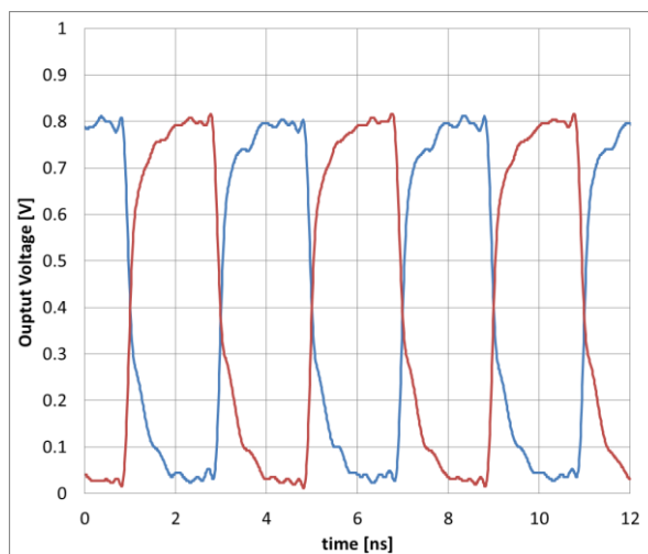
Figure 24. 250MHz HCSL
