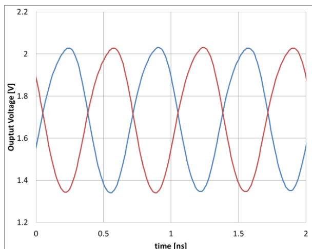
Figure 20. 1.5GHz LVPECL
