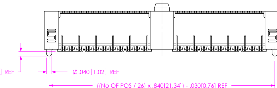
FIG 1 QFSS-052-04.25-X-D-A SHOWN
