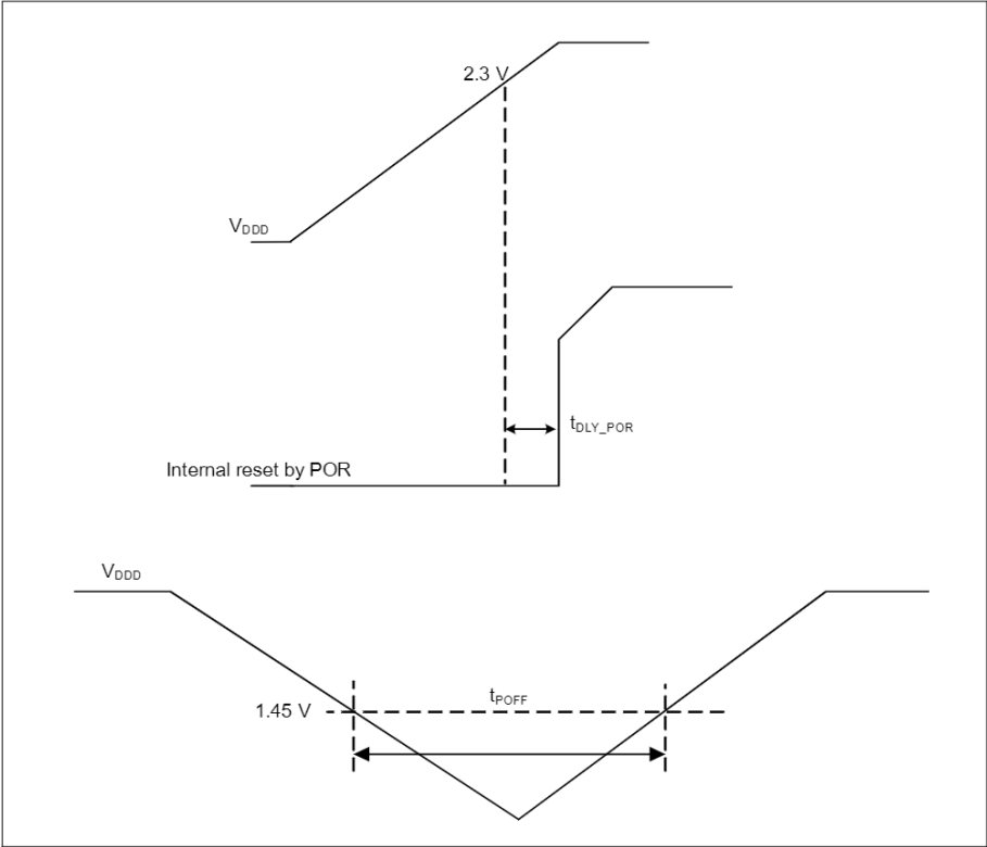
Figure 26-15 POR specifications
