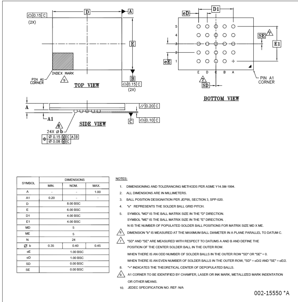
Figure 64 Ball grid array 24-ball 6 x 8 mm (VAA024)
