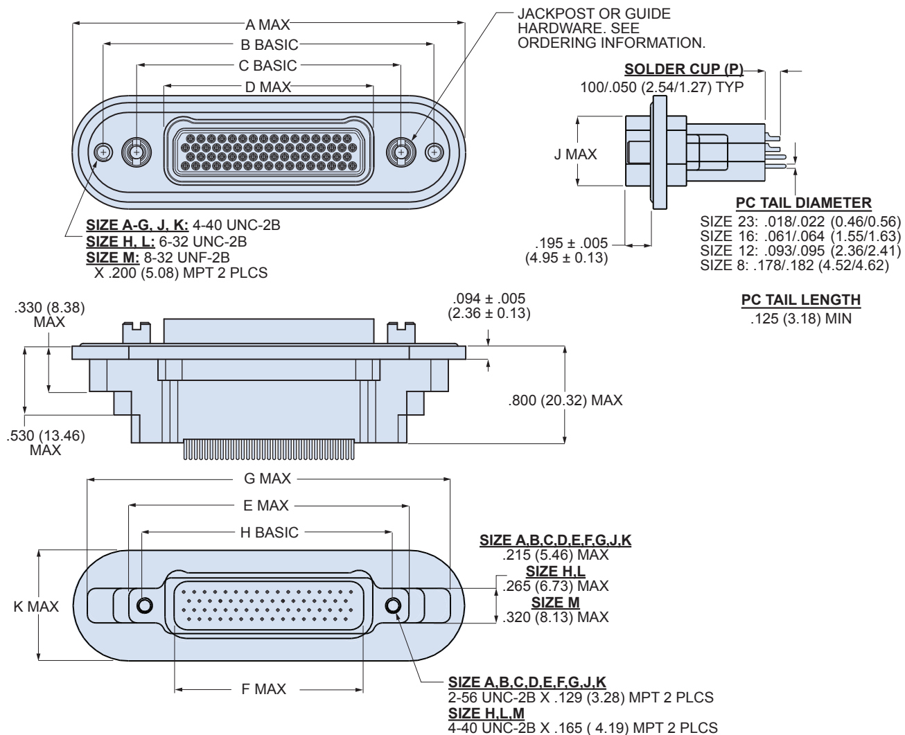
791-044 Dimensions
