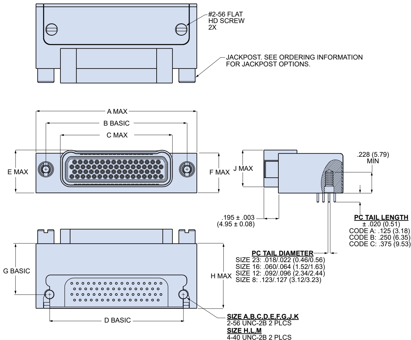
791-032P Dimensions
