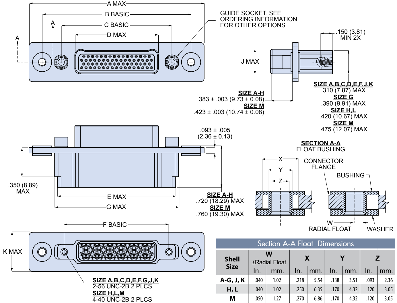
791-018S Dimensions
