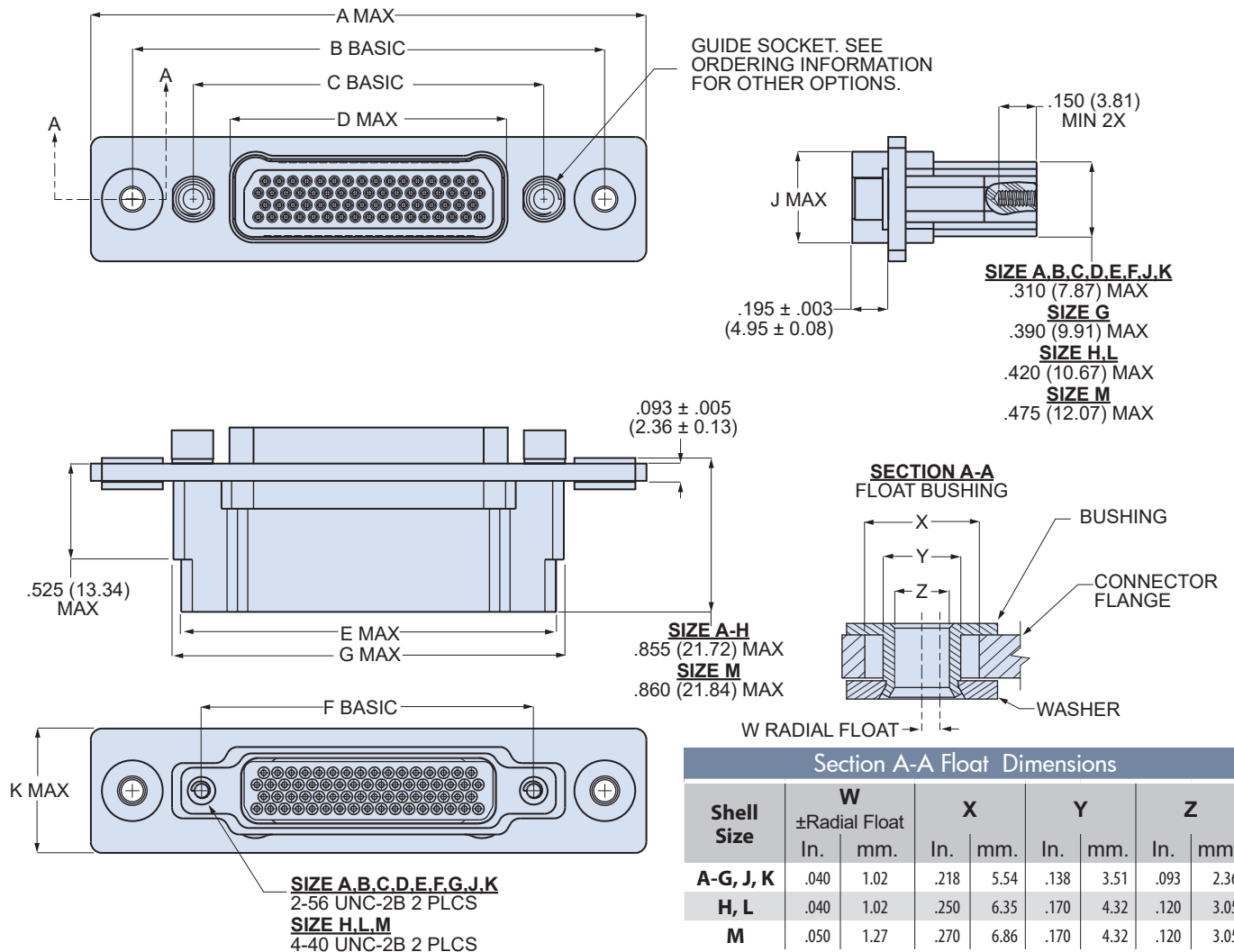
791-017P Dimensions
