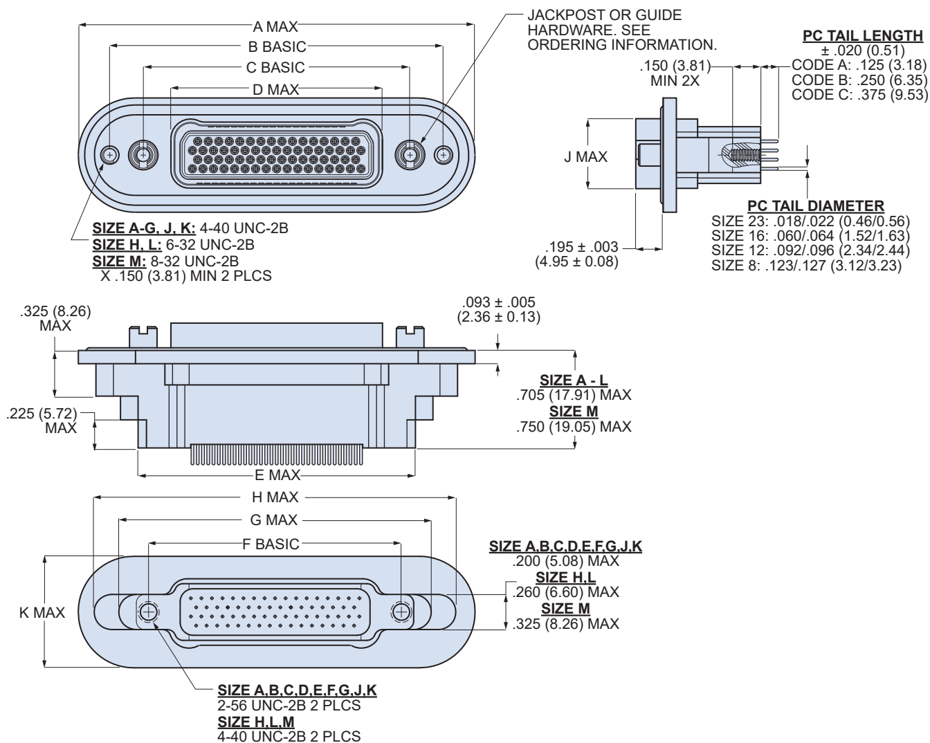
791-021P Dimensions
