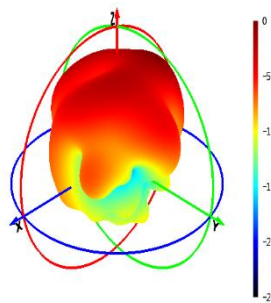
2140 MHz
