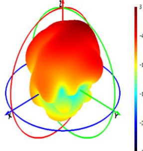
2350 MHz
