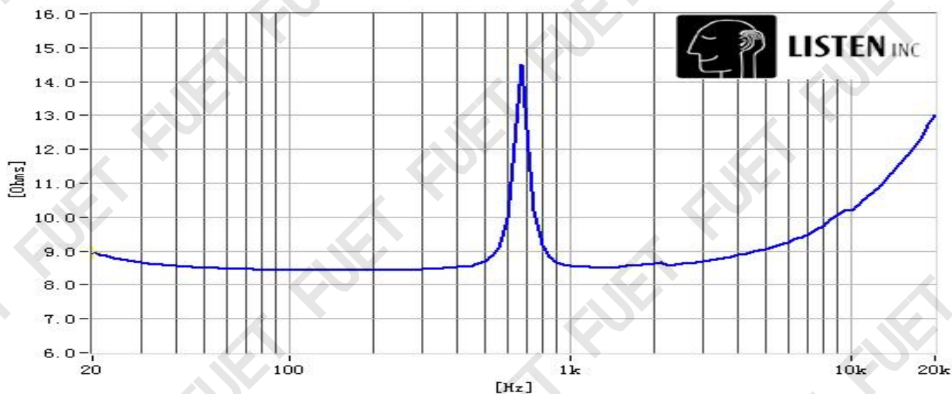
阻抗曲线
