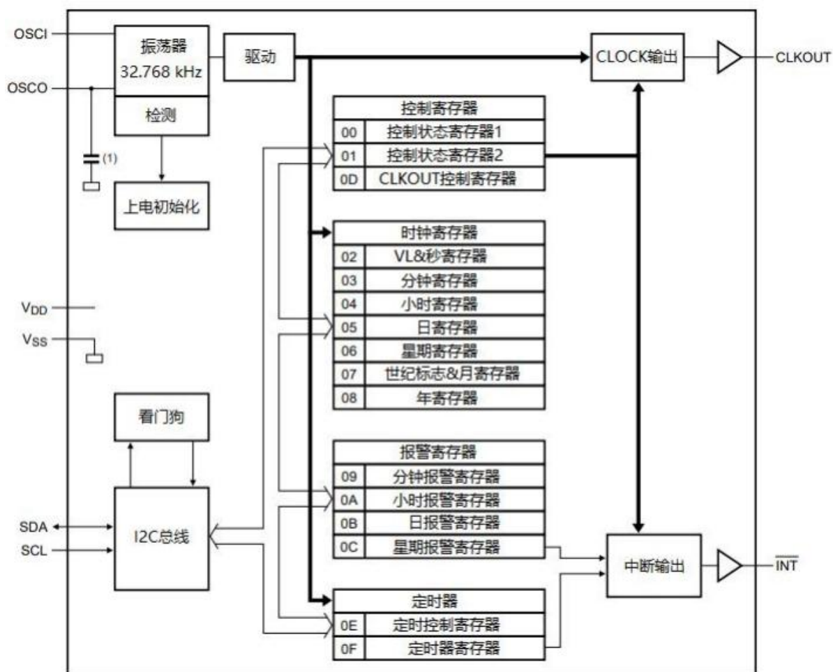
图 2. PCF85163 方框图
