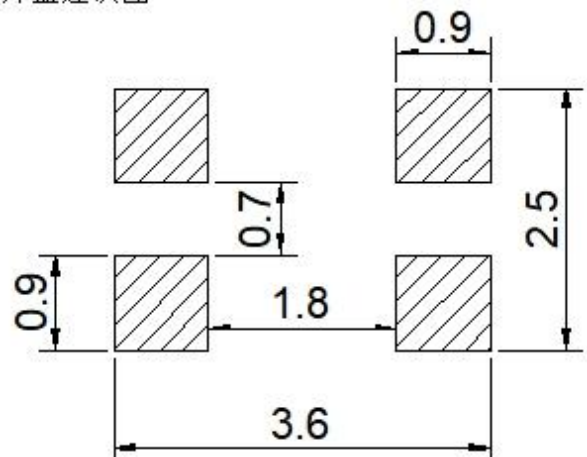
焊盘建议图
