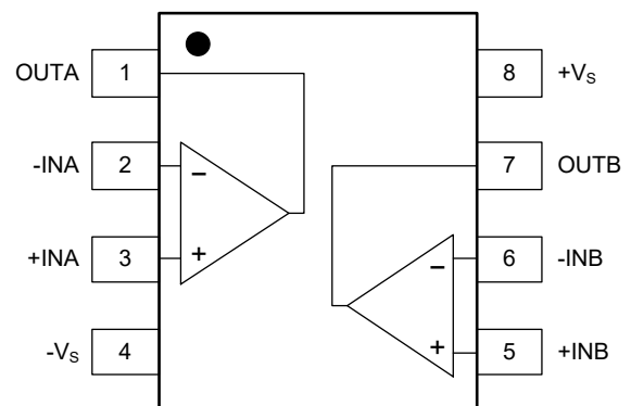
SOIC-8
