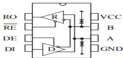
图 1 引脚分布图
