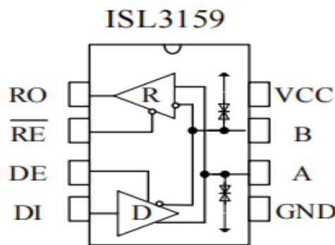
图 1 引脚分布图
