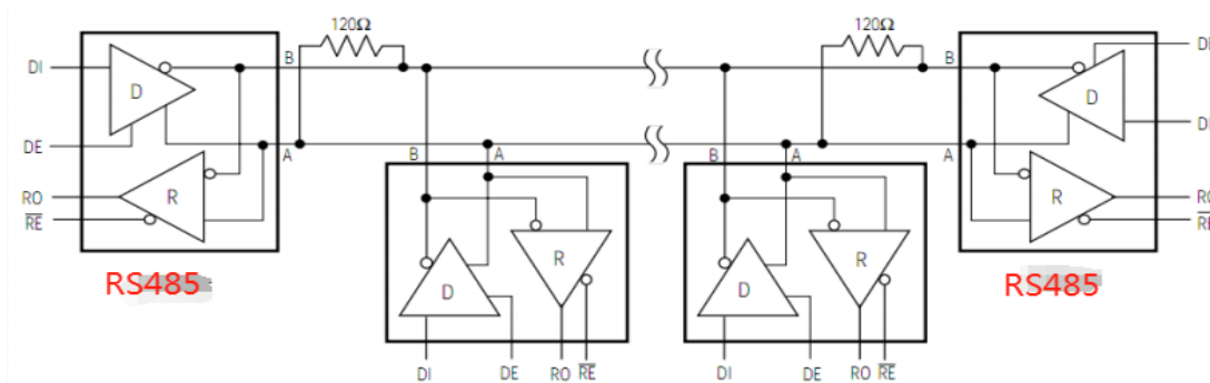
图 11 典型的 RS485 半双工通讯网络
