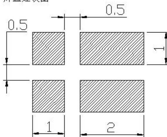
焊盘建议图
