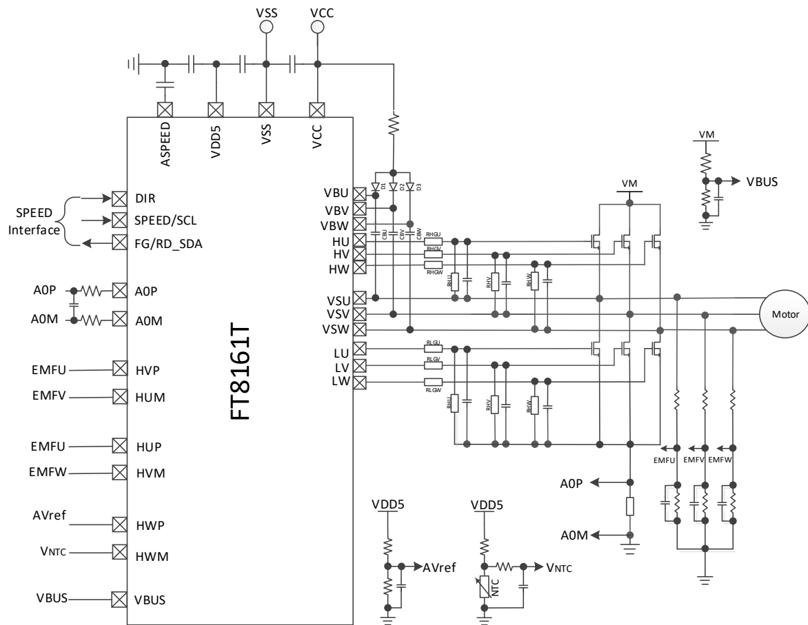
图 1-3 FT8161T 无感 FOC 单电阻应用示意图
