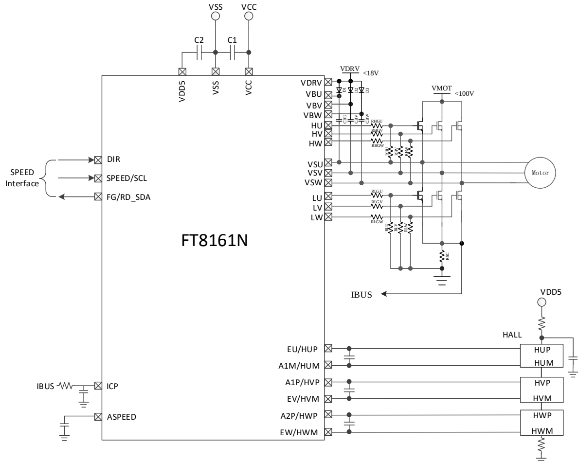
图 1-1 FT8161N 有感 SVPWM 应用示意图
