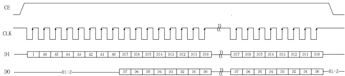
图 5.6 多字节读
