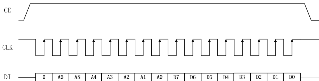
图 5.3 单字节写
