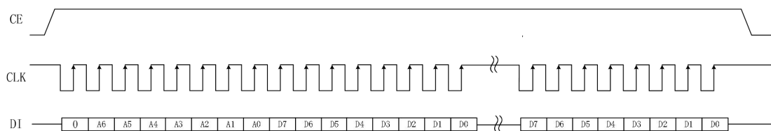
图 5.5 多字节写
