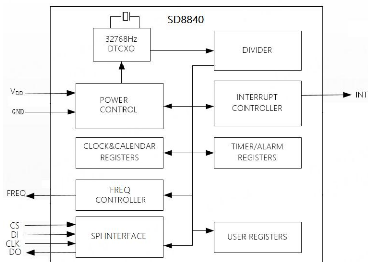
SD8840 功能框图
