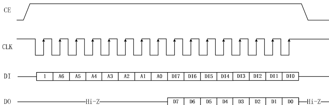
图 5.4 单字节读
