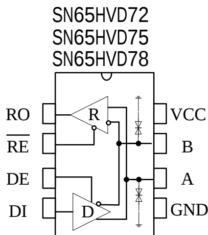
图 1 引脚分布图
