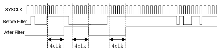
图 15-4 滤波模块时序图
