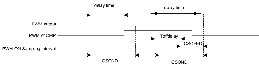
图 29-14 PWM ON 采样模式
