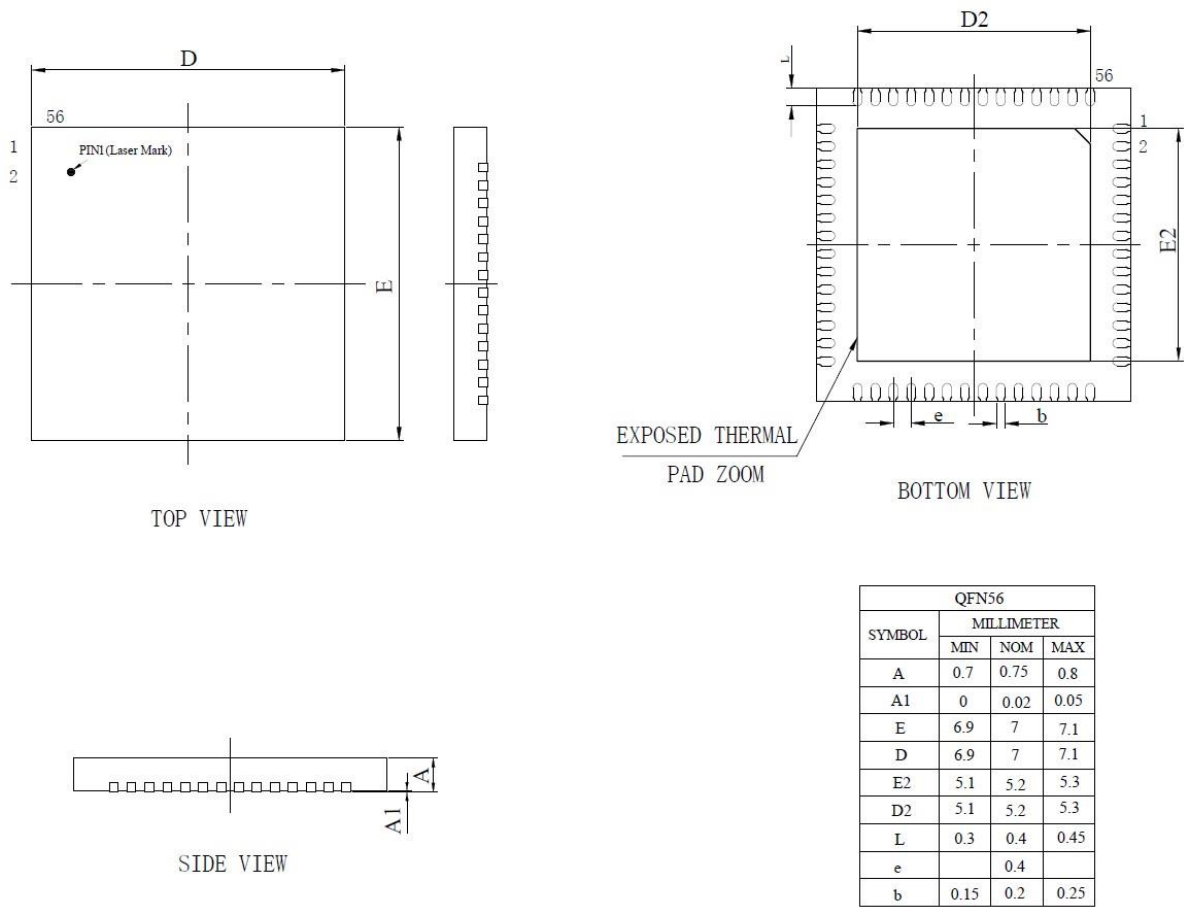
图 3-3 QFN56_7X7 封装尺寸图
