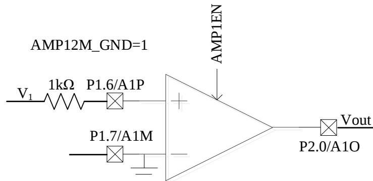
图 28-9 AMP1 工作在 PGA 单端输入模式
