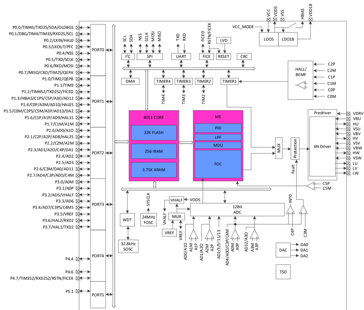
图 1-3 FU6865Q 功能框图
