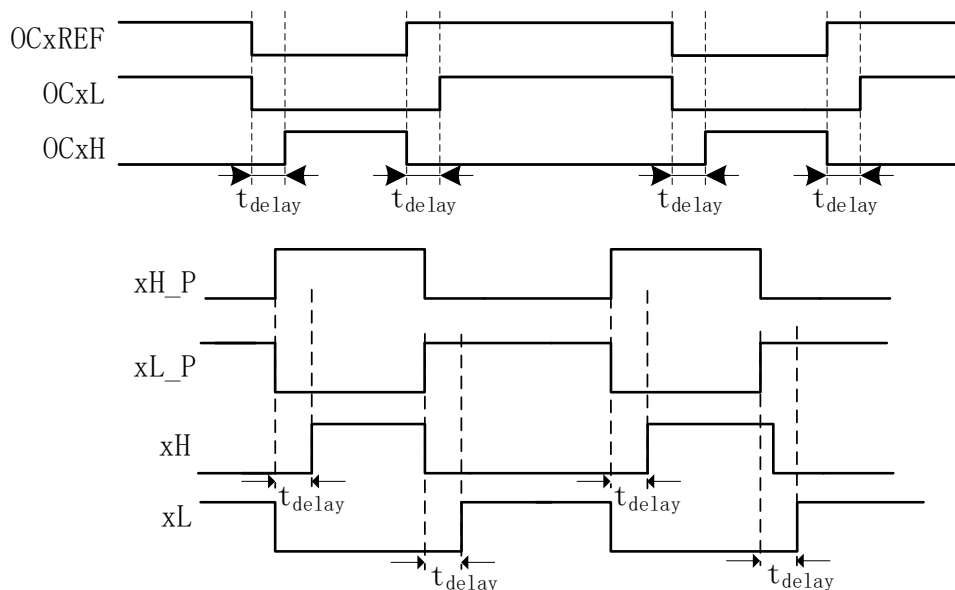
图 18-5 带死区插入的互补输出
