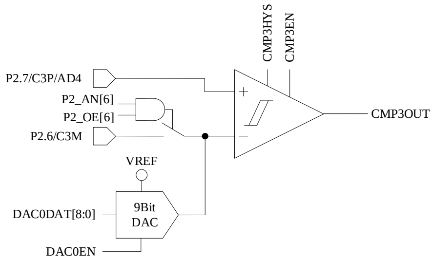
图 29-2 单比较器输入模式
