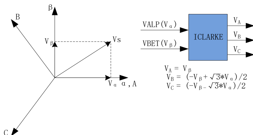
图 13-3 Clarke 逆变换
