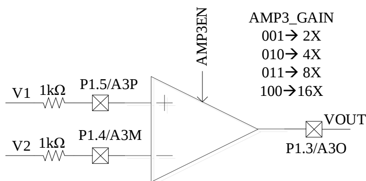
图 28-12 AMP3 工作在 PGA 差分输入模式
