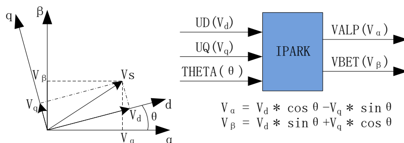
图 13-2 Park 逆变换
