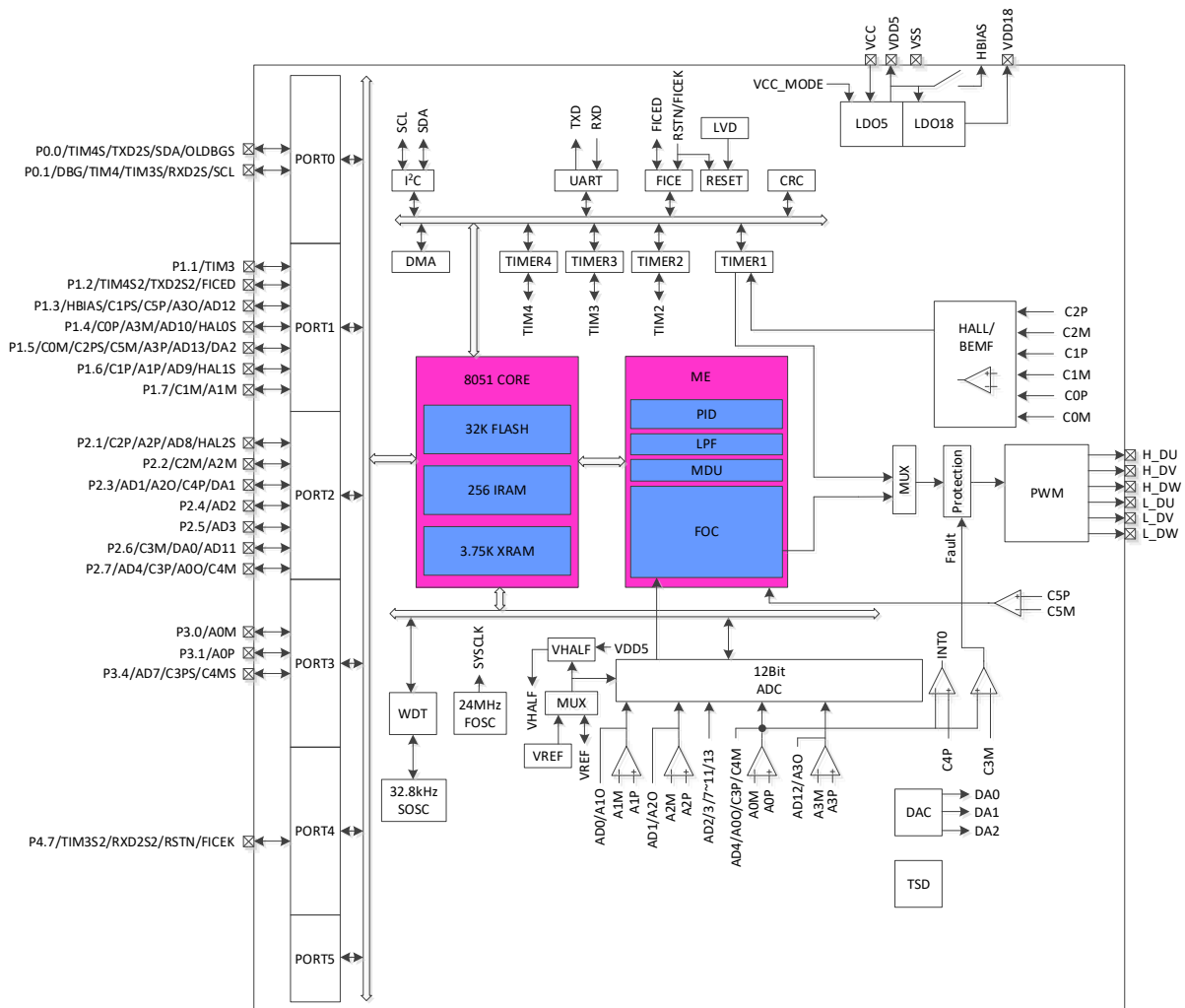
图 1-2 FU6815T 功能框图
