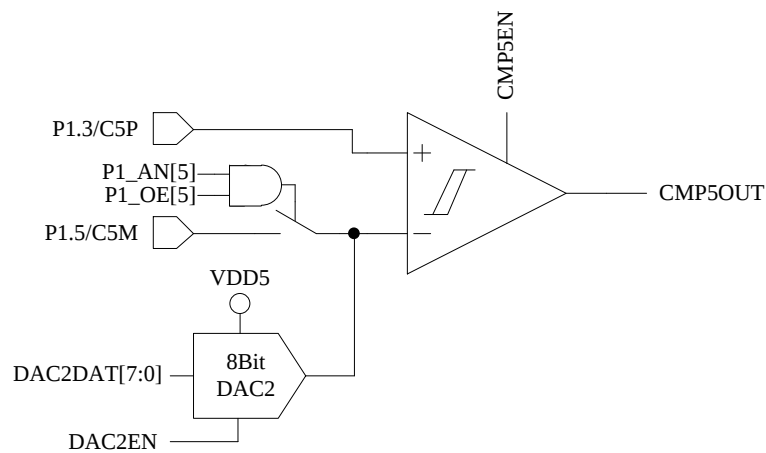
图 29-8 CMP5 模块示意图
