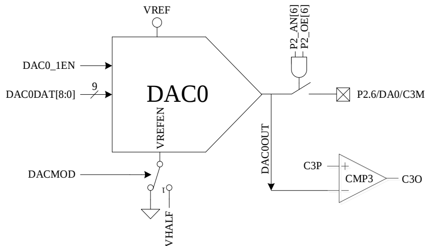
图 24-1 DAC0 功能框图
