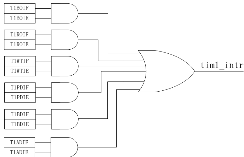
图 14-10 Timer1 中断源
