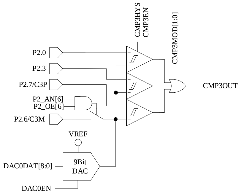
图 29-4 三比较器输入模式
