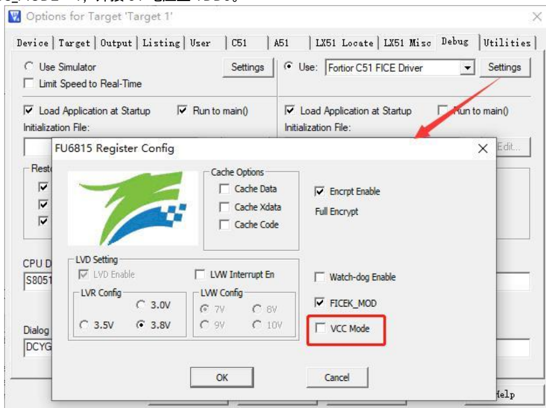
图 30-2 VCC_MODE 配置
