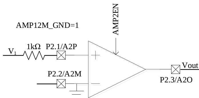
图 28-10 AMP2 工作在 PGA 单端输入模式
