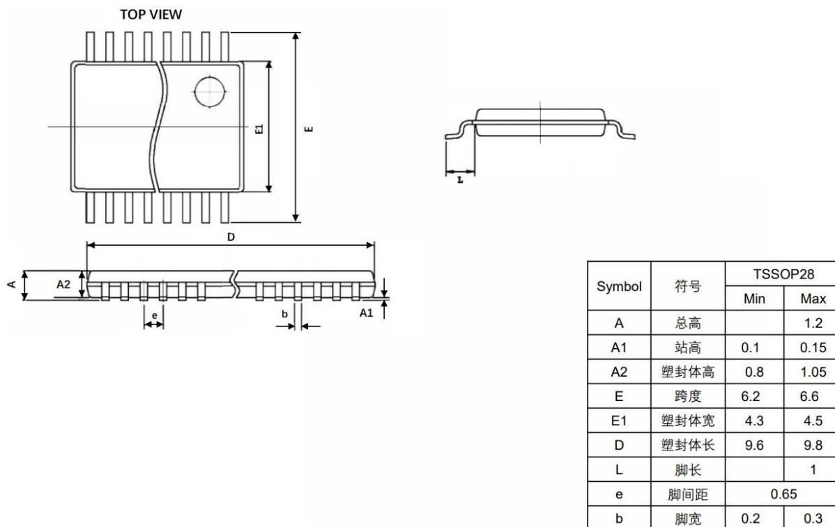
图 3-2 TSSOP28_9.7X4.4 封装尺寸图
