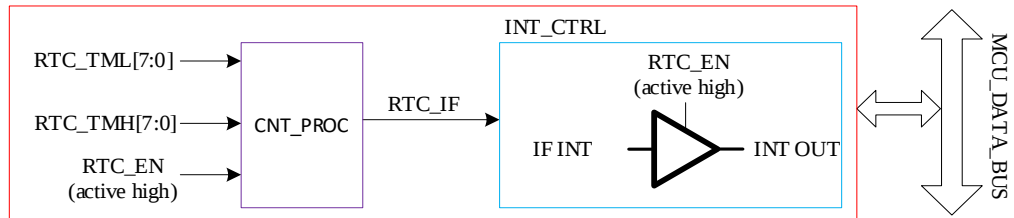
图 21-1RTC 基本功能框图
