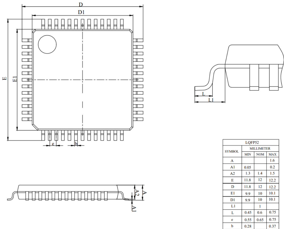
图 3-5 LQFP52_10X10 封装尺寸图
