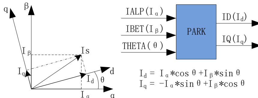
图 13-5 Park 变换
