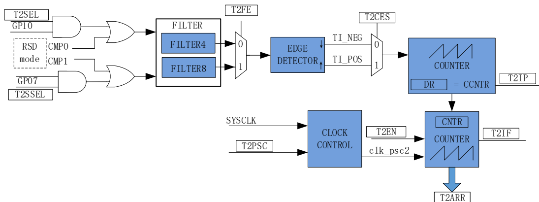
图 15-7 输入计数模式原理框图
