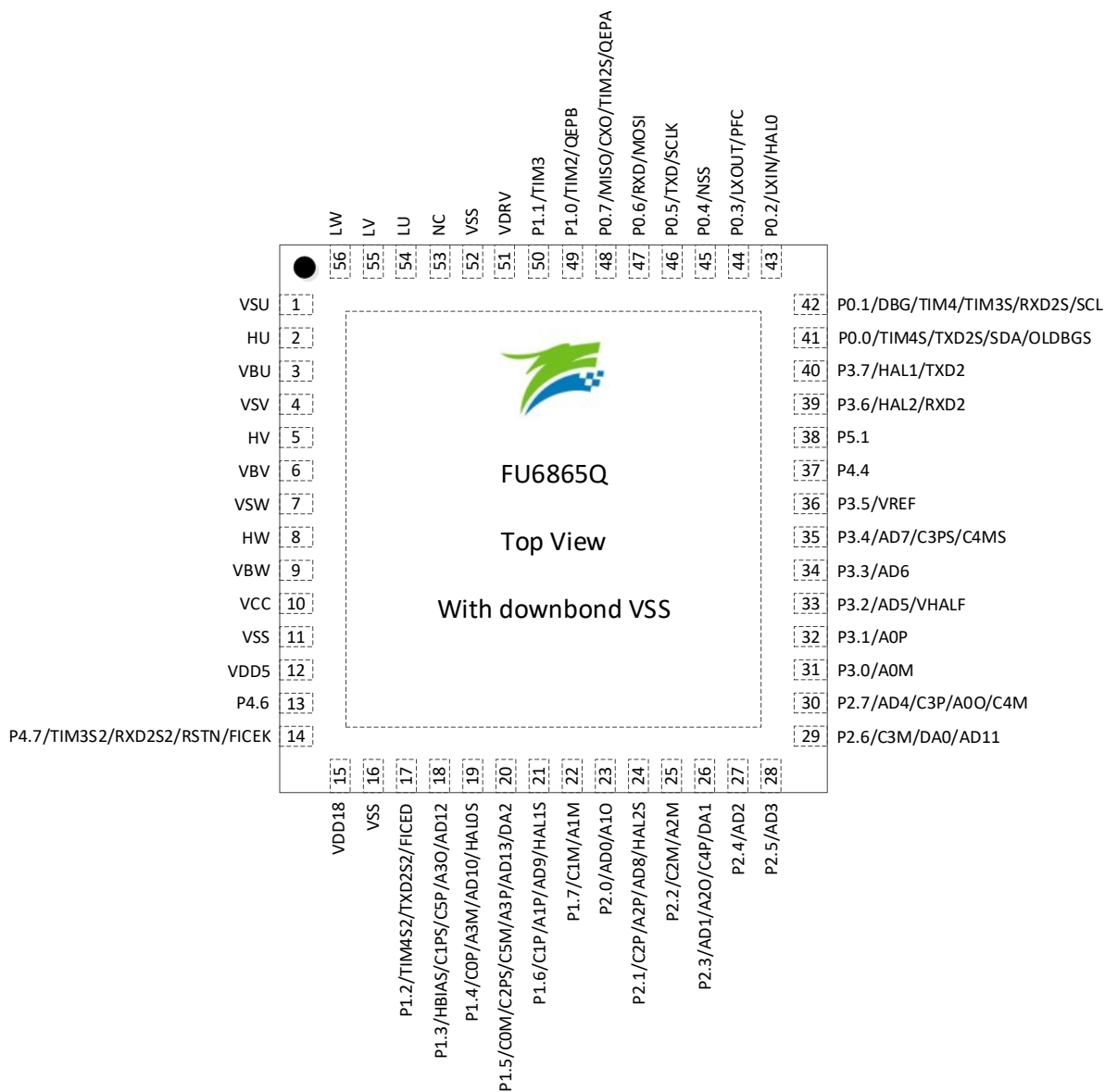
图 2-3 FU6865Q QFN56 引脚图
