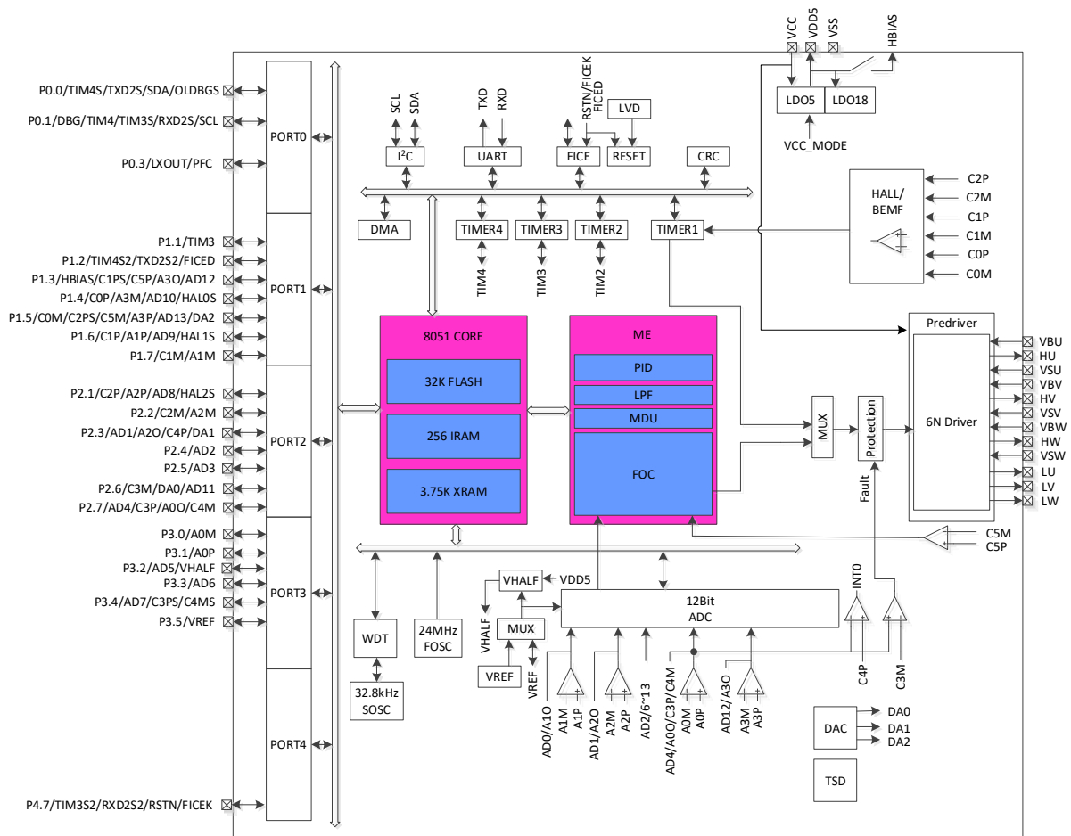
图 1-5 FU6864L 功能框图
