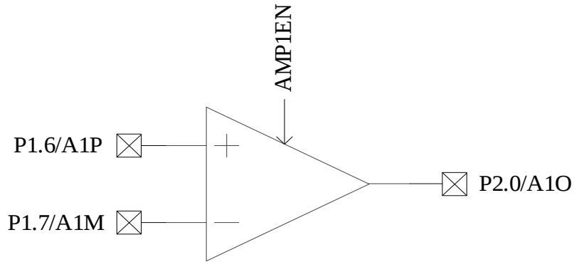
图 28-5 AMP1 输入输出相关端口
