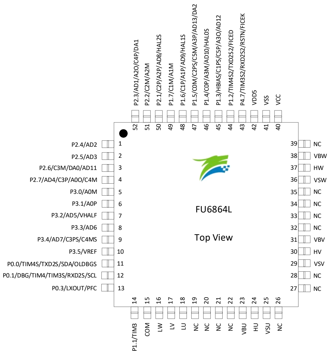
图 2-5 FU6864L LQFP52 引脚图
