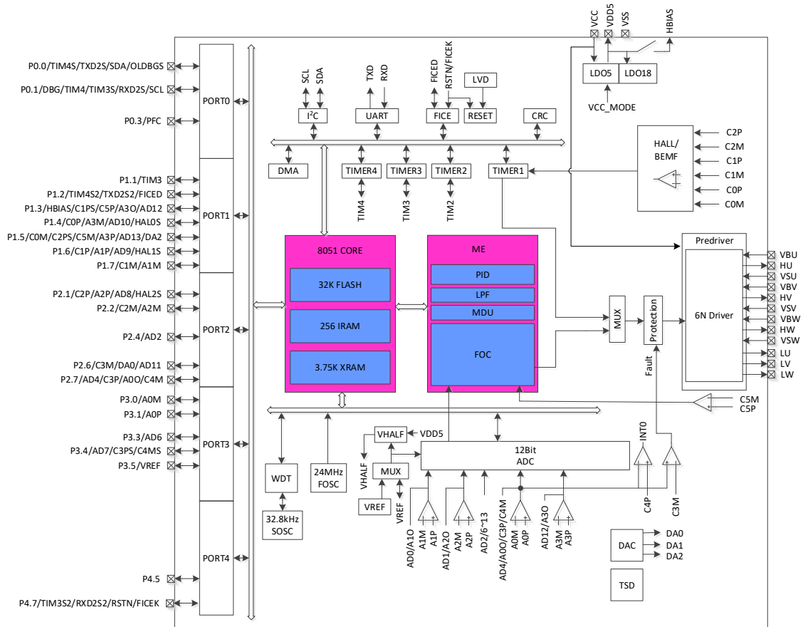
图 1-4 FU6864Q 功能框图
