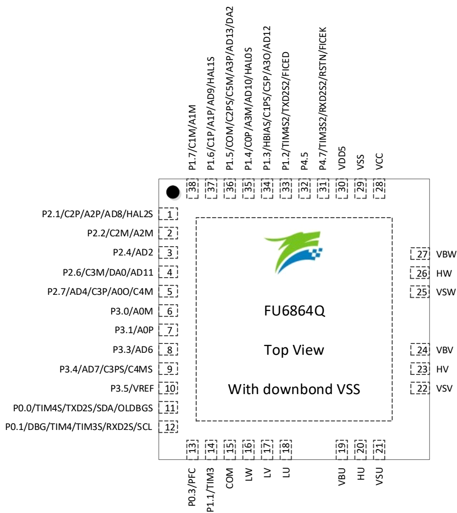
图 2-4 FU6864Q QFN48-38 引脚图
