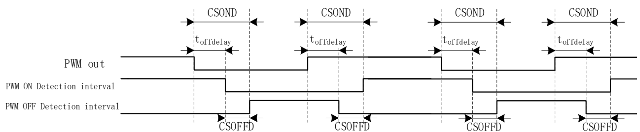
图 14-7 采样区间图
