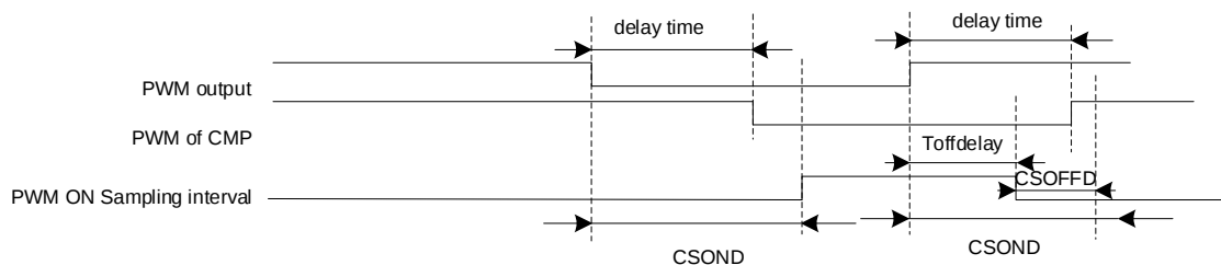
图 29-15 PWM OFF 采样模式
