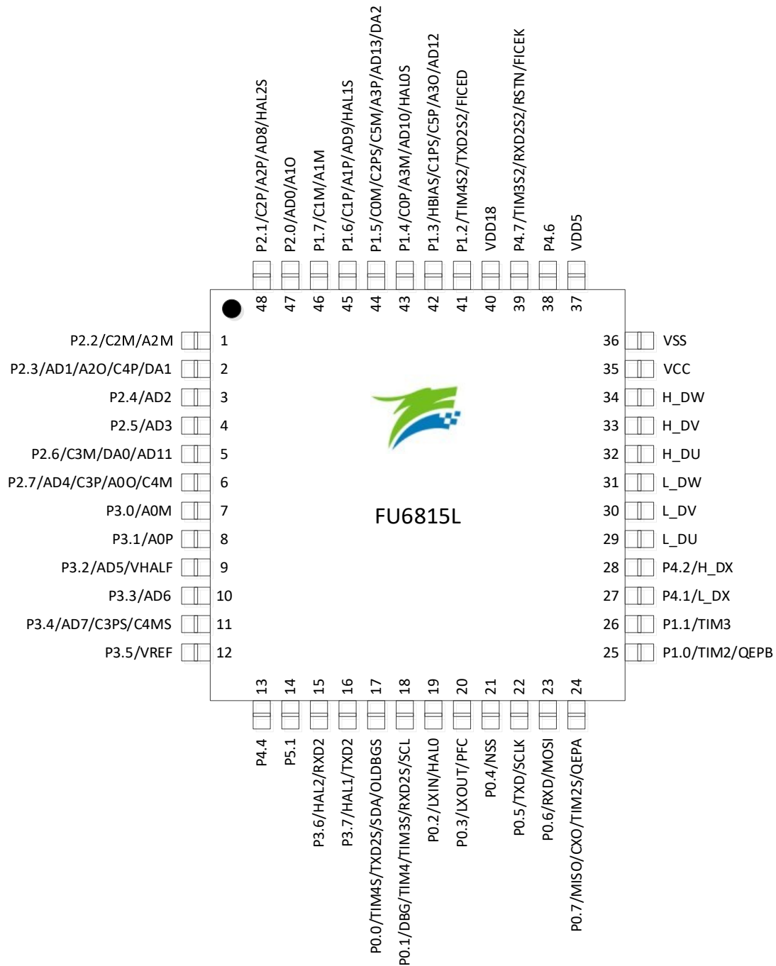
图 2-1 FU6815L LQFP48 引脚图
