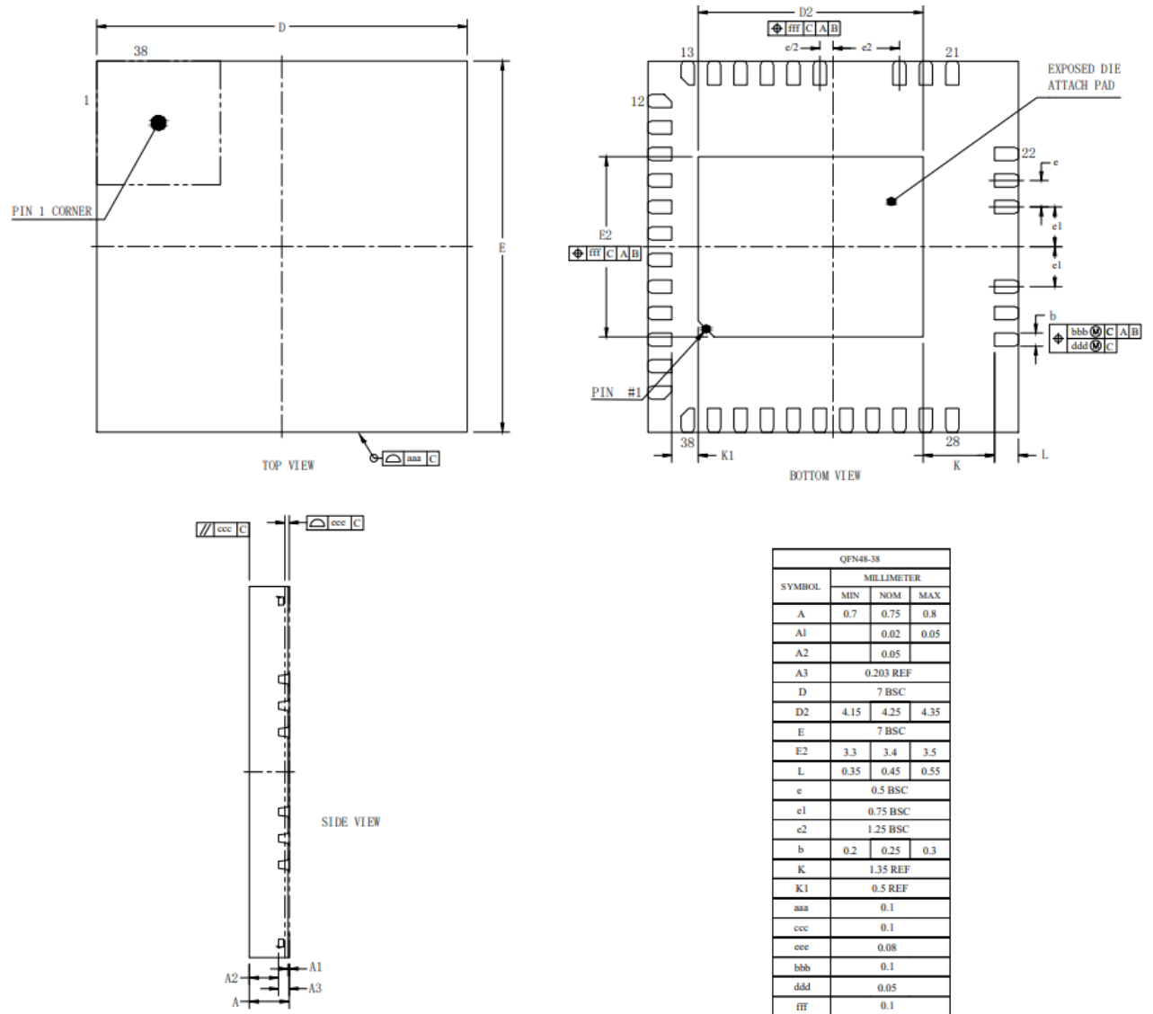
图 3-4 QFN48-38_7X7 封装尺寸图
