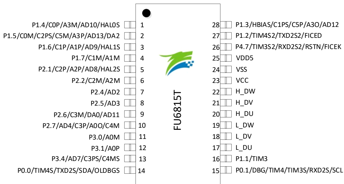
图 2-2 FU6815T TSSOP28 引脚图
