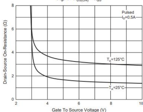
Fig. 4 - R_{DS(ON)} - V_{GS}
