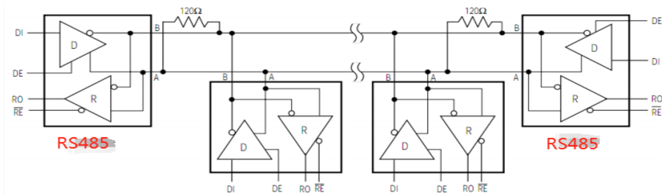
图 11 典型的 RS485 半双工通讯网络
