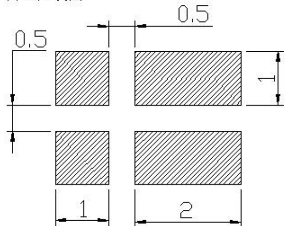
焊盘建议图
