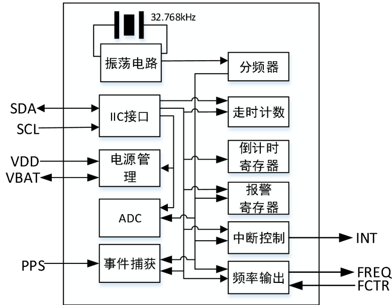
功能框图
